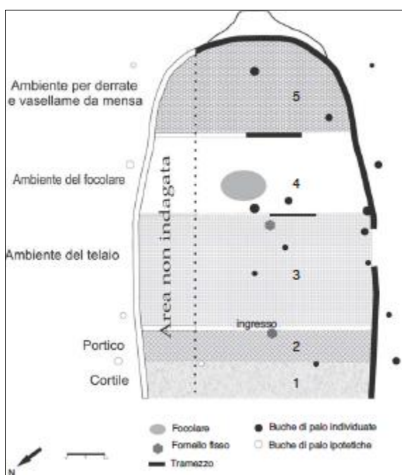
Fig. 2 Planimetria con indicazione delle aree funzionali della dimora absidata, Torre di Satriano (da CAROLLO 2009, p. 20, fig. 1)
