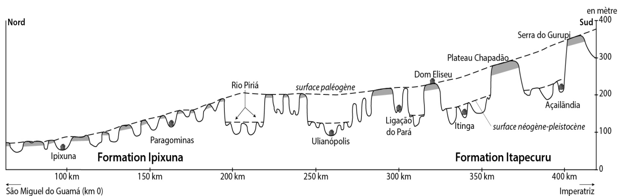
Figure 27. Schéma topographique régional le long de la route BR-010 d'après (Kotschoubey et al. 2005)
