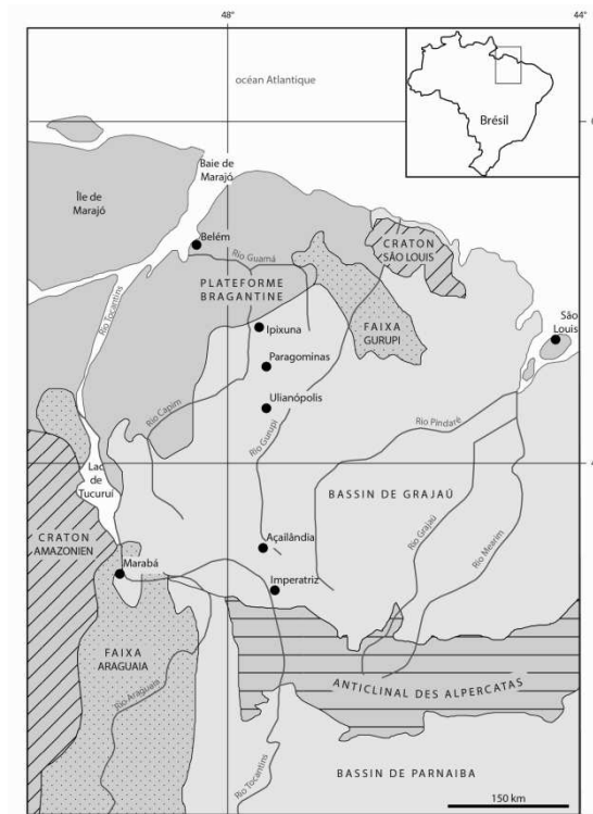
Figure 25. Contexte géologique régional, d'après (Kotschoubey et al. 2005) (In (Laurent, Pocard-Chapuis, et al. 2017)
