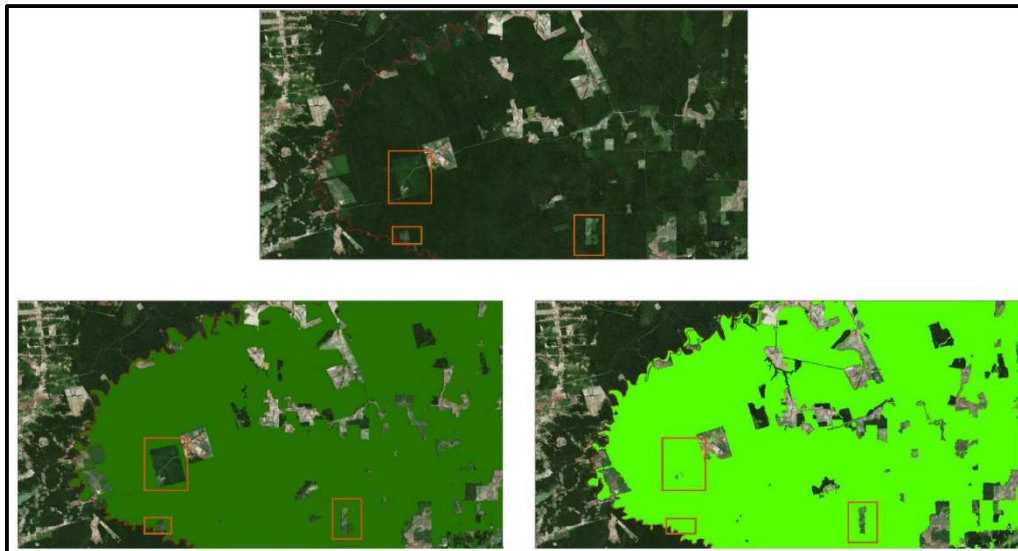
Figure 39. Comparaison de l'image Esri "World Imagery" (en haut) avec le masque pluriannuel PALSAR/PALSAR-2 (en bas à gauche) et le masque pluriannuel de forêt primaire résultant de la classification orientée objet CLASlite (en bas à droite). Les rectangles orange représentent les zones de pâturages dégradés ou les zones de forêts secondaires visibles avec ESRI "World Imagery", non masquées par PALSAR / PALSAR-2 mais masquées avec la classification CLASlite.
