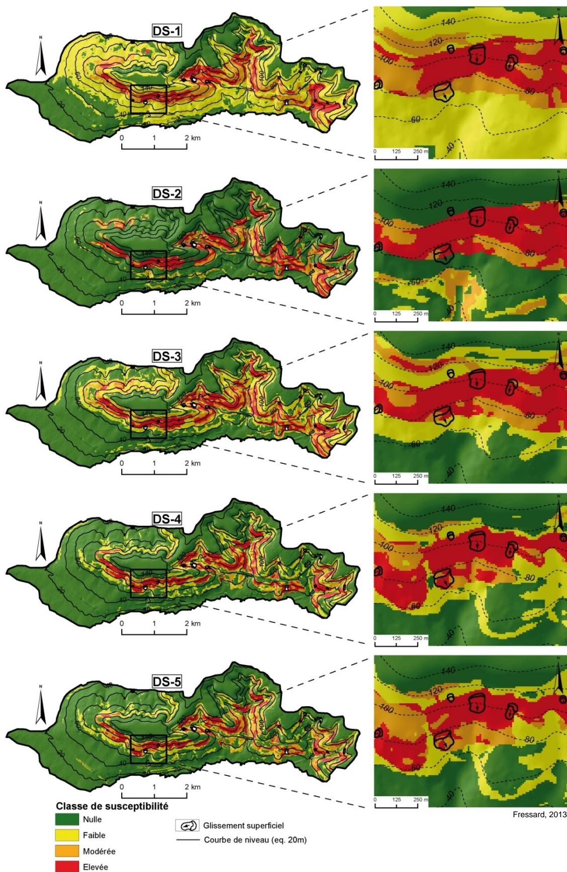
Figure 7.19 : Cartes de susceptibilité finales modélisées par régression logistique pour chacun des sets de données collectées et zoom illustratif
