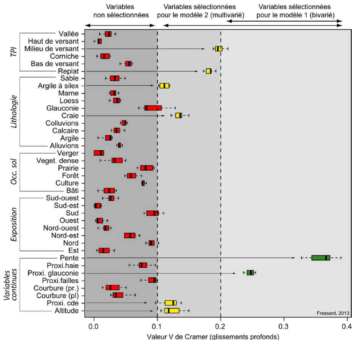
Figure 7.4 : Diagramme en boîtes des résultats de l'itération répétée (n=10) du test du V de Cramer visant à tester l'association entre la localisation des glissements profonds et les variables sélectionnées
