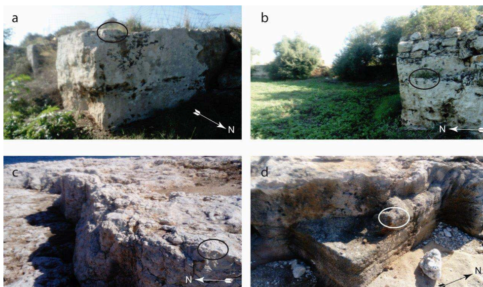
a) Intagliata, fronts Nord-Ouest ; b) Intagliata, fronts Est ; c) Thapsos 1, fronts supérieurs Sud ; d) Thapsos 3, fronts Sud-Ouest. Clichés F. Mège.
