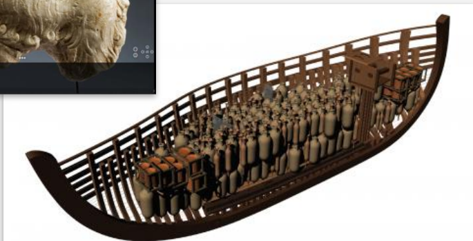
Vue de 3/4 du modèle 3D de restitution du flanc tribord et de la cargaison du Dramont E. (P. Poveda CNRS-CCJ)
