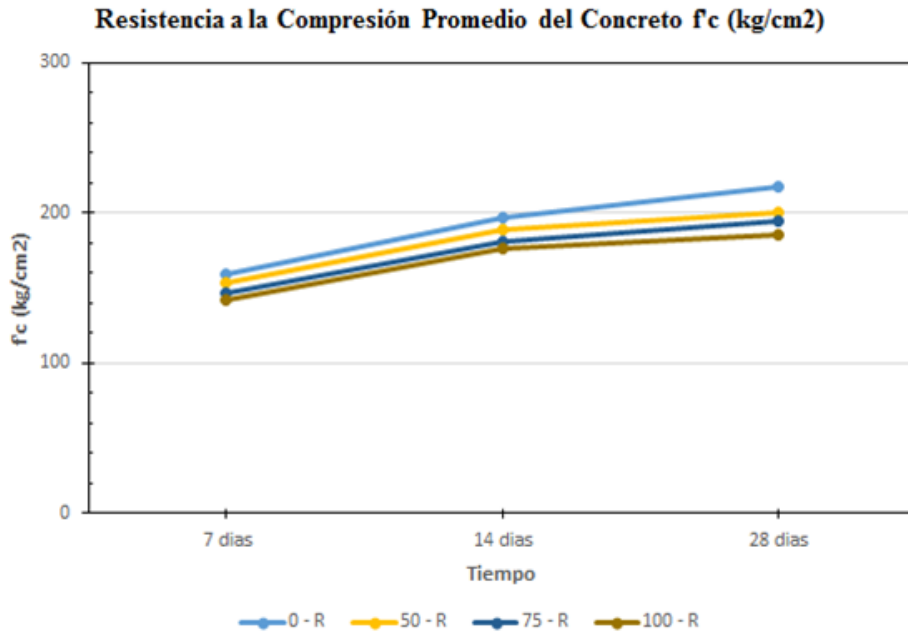
Figura 2. Resistencia a la compresión promedio del concreto convencional y del concreto de agregados reciclados.
