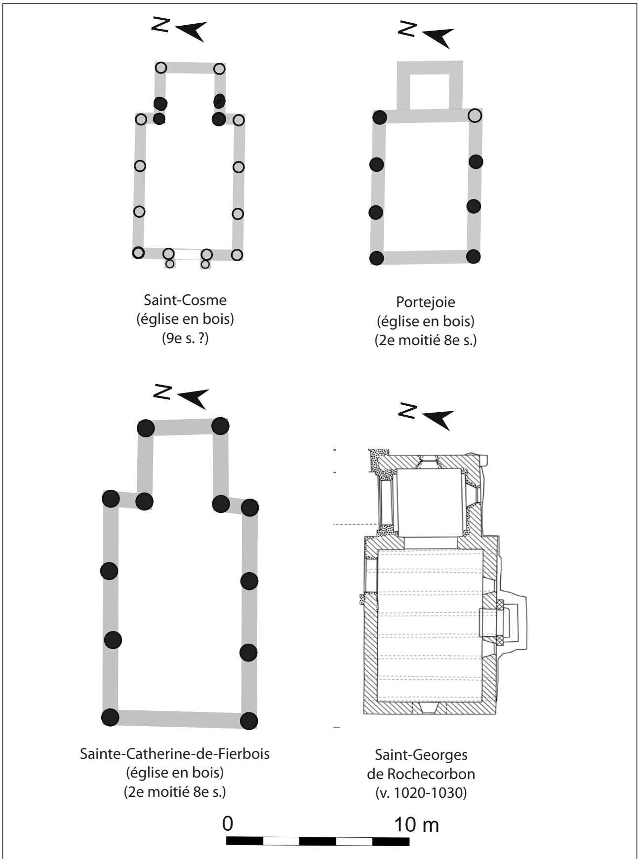
Figure 14 bis : comparaison entre l'église à poteaux de bois de Saint-Cosme et d'autres églises
