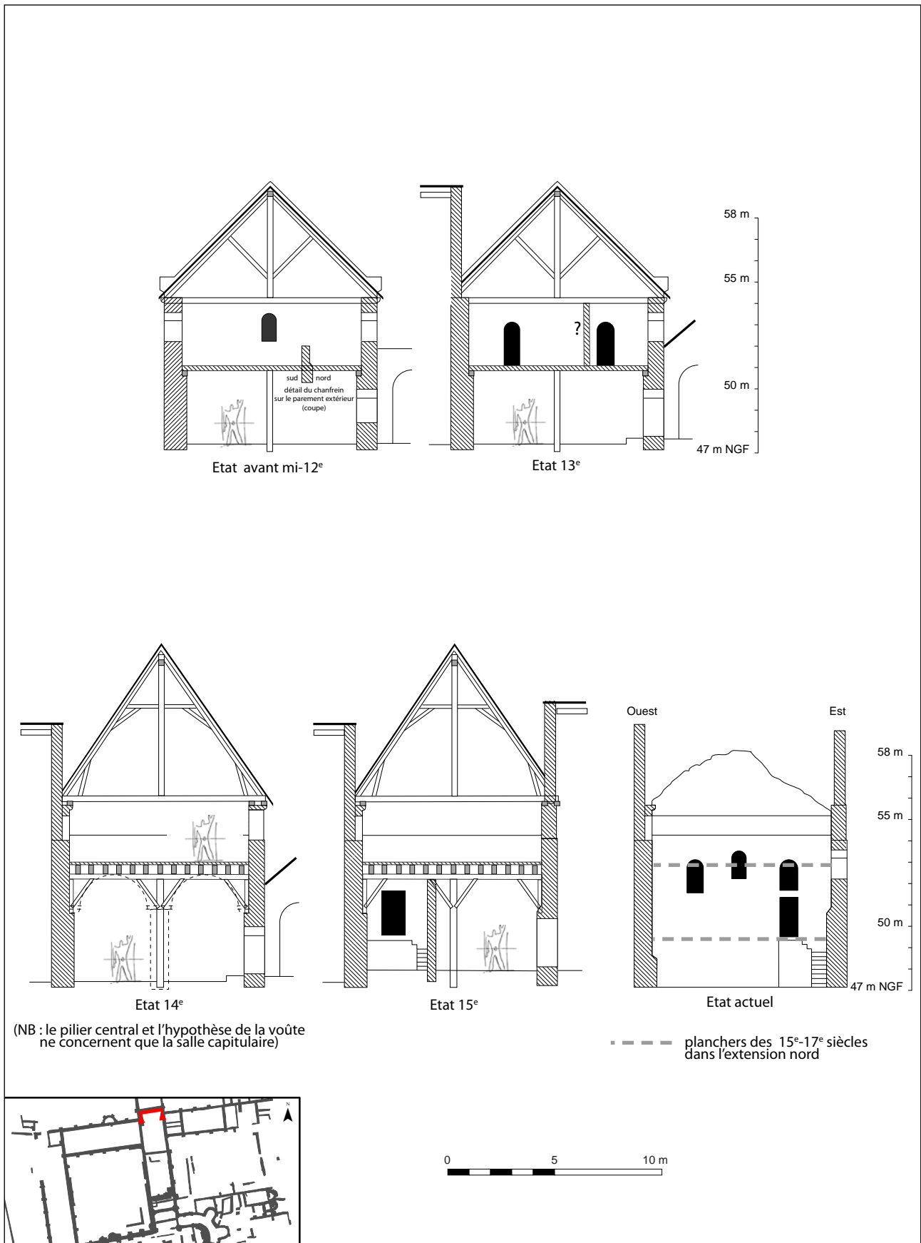
Figure 38 : restitution phasée de l'élévation de l'aile orientale du carré claustral (coupes est-ouest à son extrémité nord)
