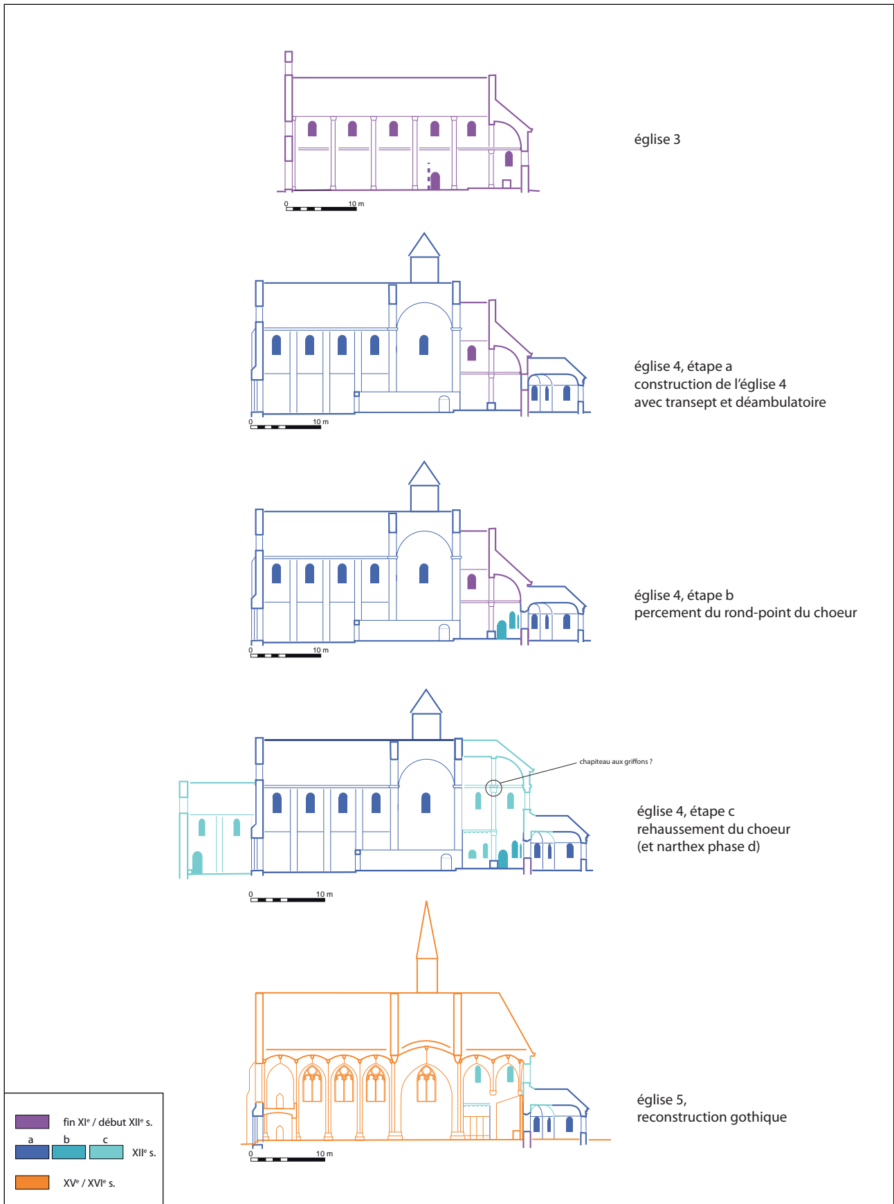
Figure 20 : coupes élévations restituées des églises n°3, 4 et 5
