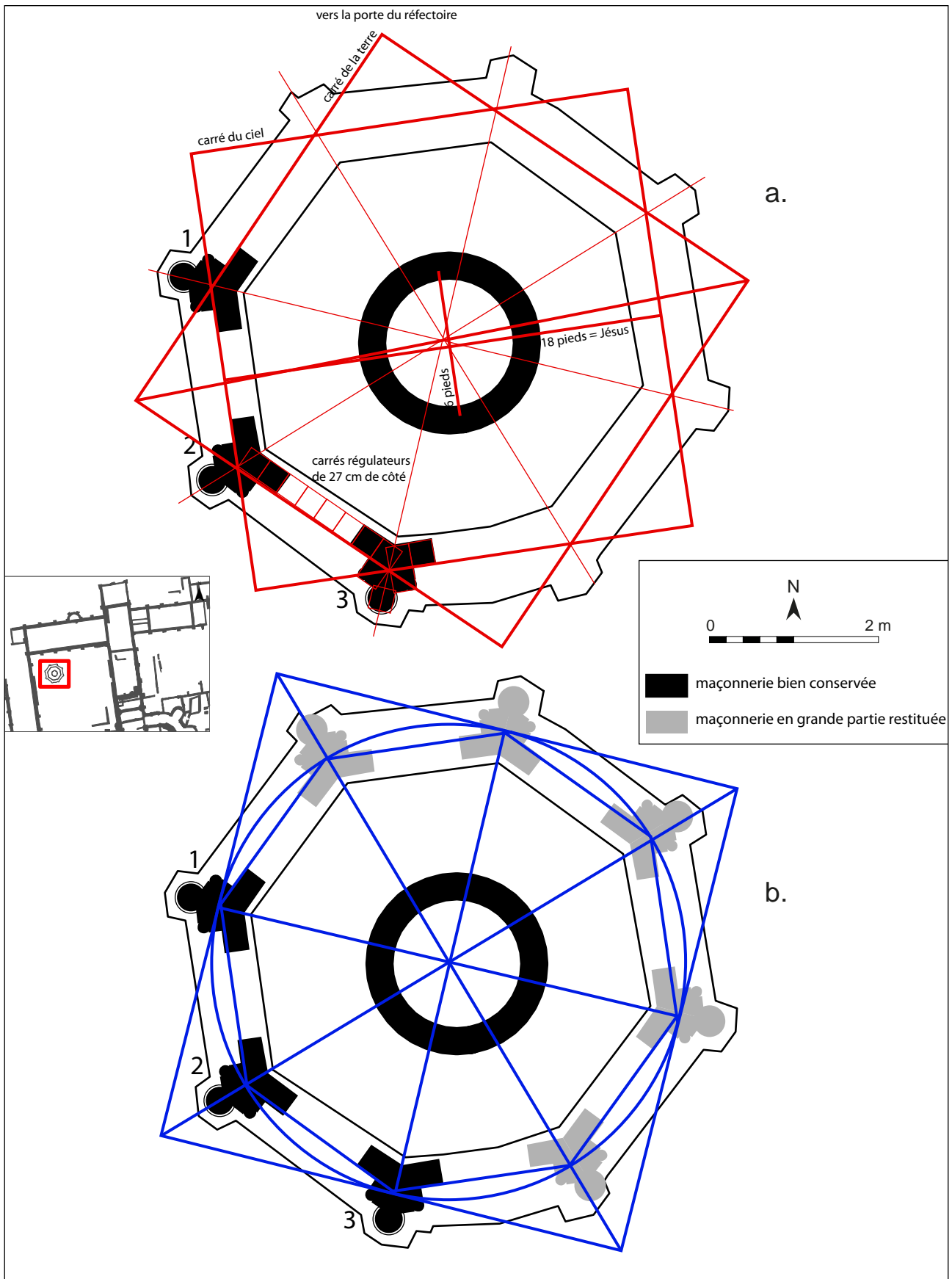
Figure 47 : a - proposition de restitution du tracé régulateur de l'octogone du lavabo du cloître b - tracé régulateur de l'octogone selon la méthode moderne
