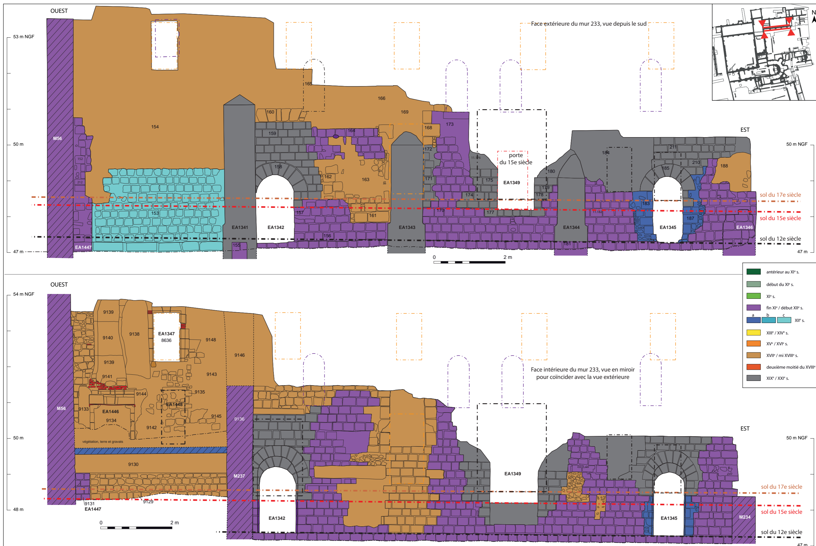
Planche 30 : analyse du bâti du mur gouttereau sud du « régulier » (M 233) (d'après le relevé de Bancaud, Body 2006, complété par Julien Noblet en 2010) – le parement interne est vu en miroir pour coïncider avec la vue extérieure
