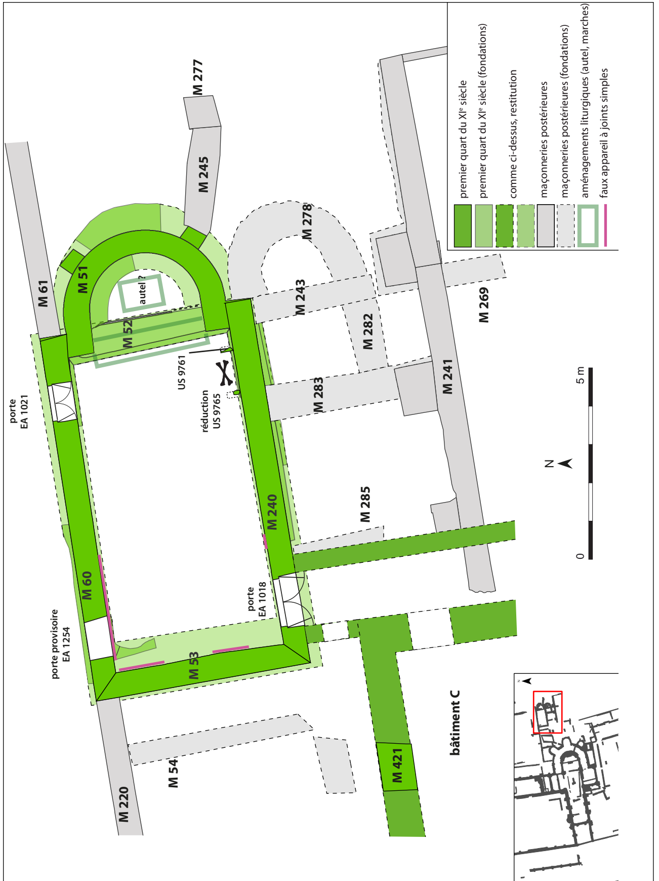
Figure 16 : plan de l'église n°2
