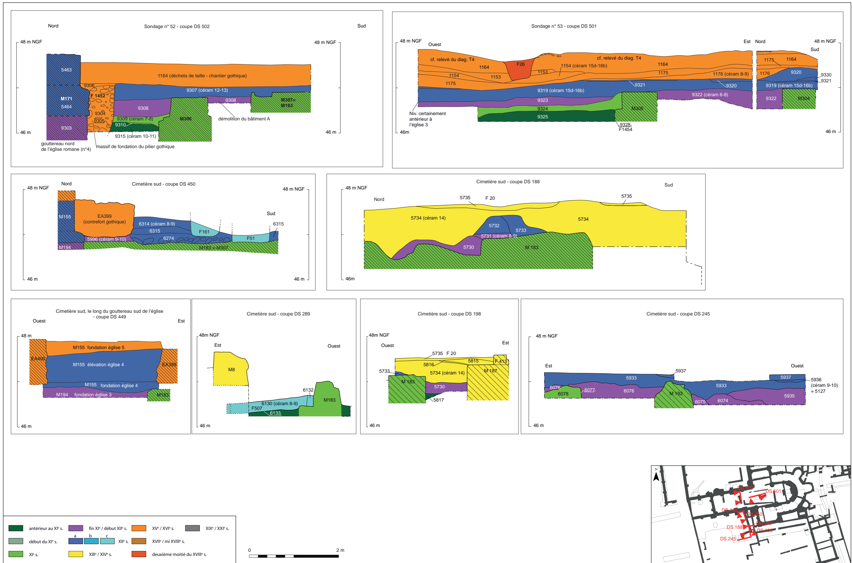
Planche 16 : coupes sur les fondations des bâtiments du 11e siècle (bâtiment A et B)
