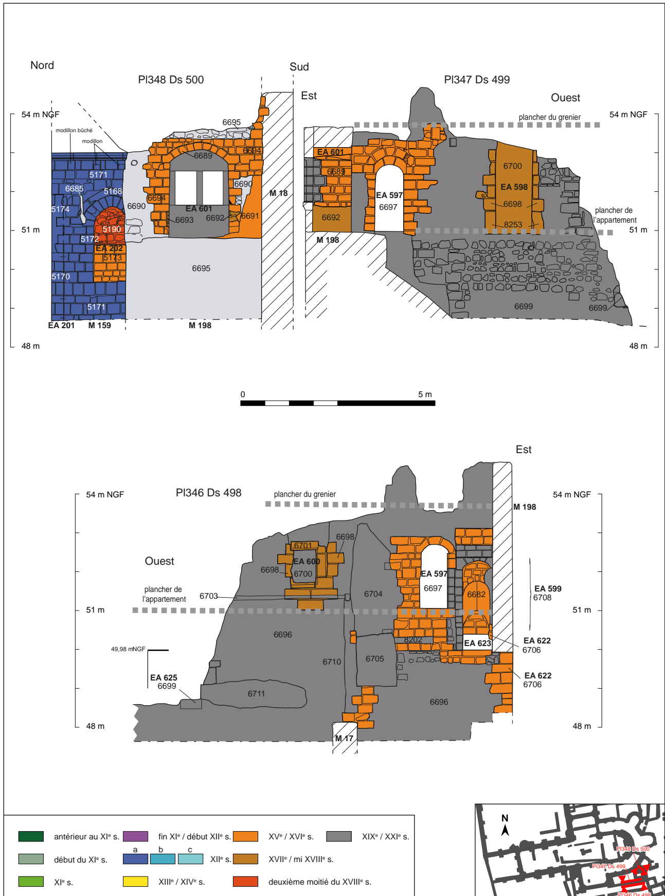
Figure 58 : élévations du mur sud (M 18) et du mur est (parement interne de M 198) du logis du sacristain jouxtant l'église au sud
