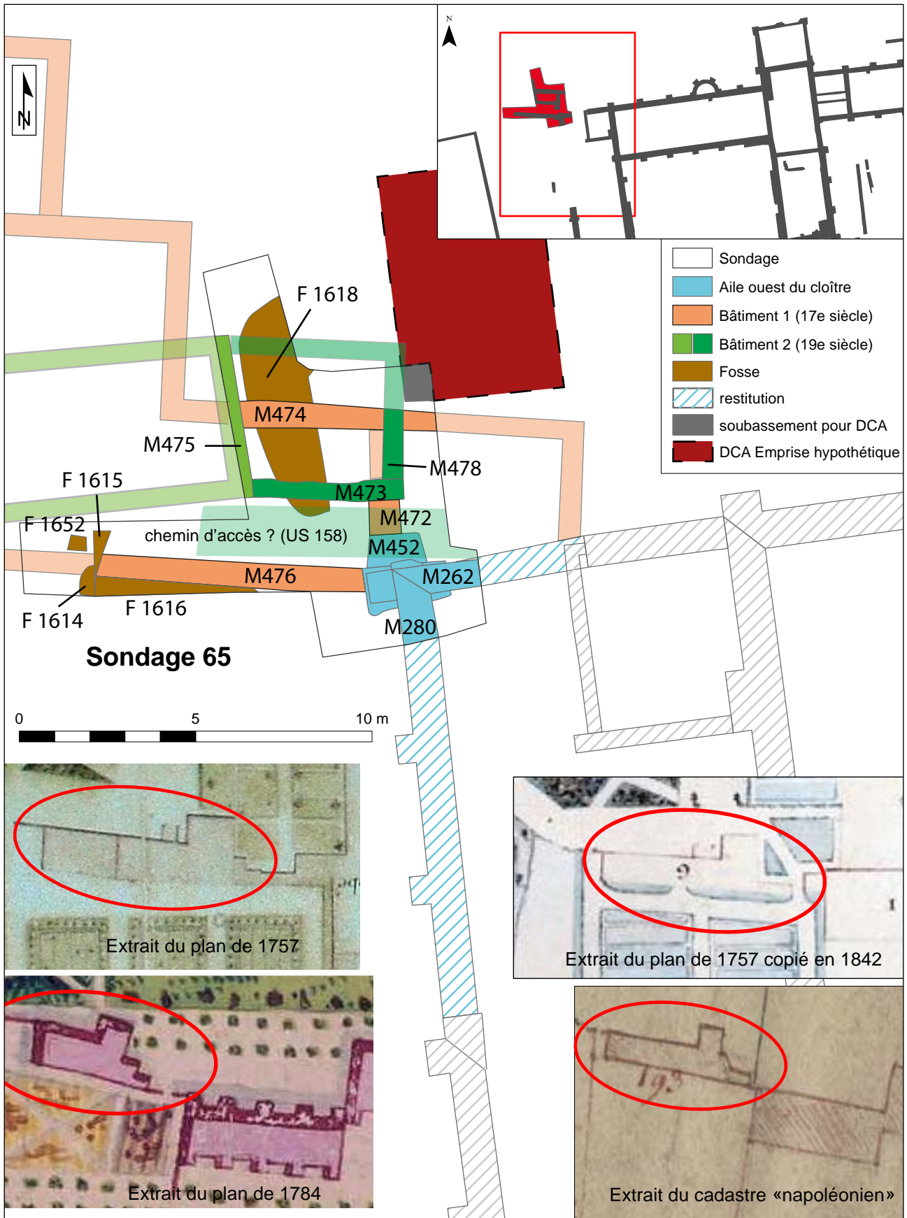
Figure 67 : plan phasé des maçonneries retrouvées en 2013 dans le sondage n°65 (logis du sacristain)
