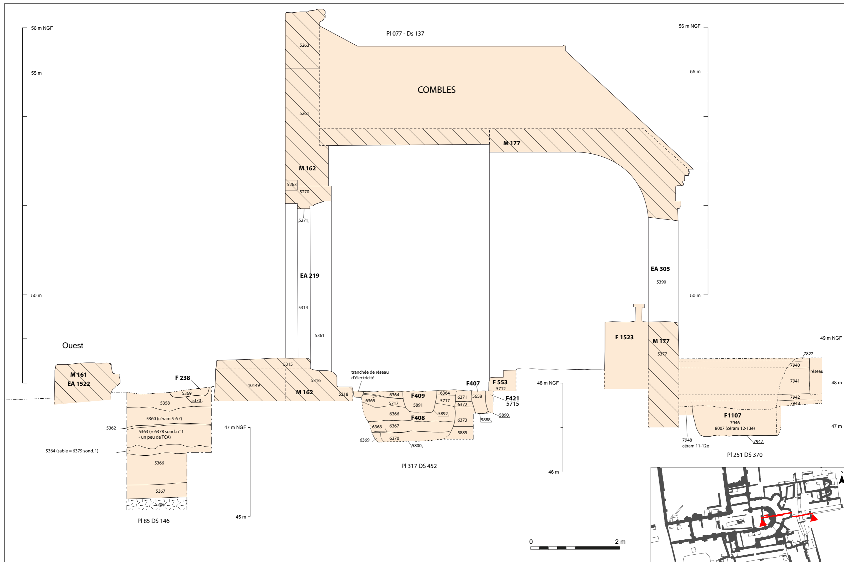
Planche 25 bis : coupe sur la chapelle axiale du déambulatoire (pour le relevé phasé, voir figure 29)
