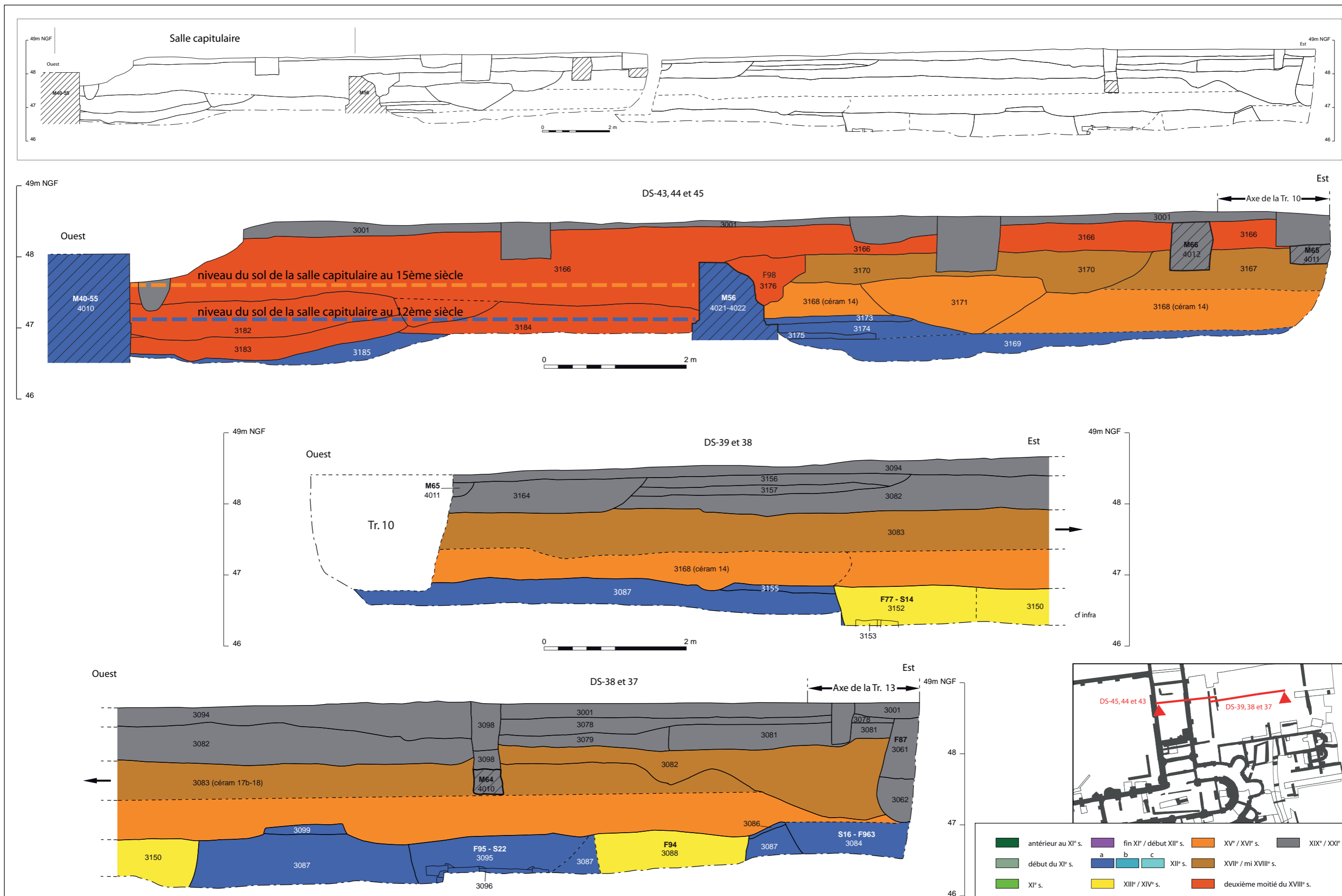
Planche 28 : analyse stratigraphique de la tranchée n°8 du diagnostic de 2006 au travers de l'aile orientale du carré claustral et du cimetière des moines
