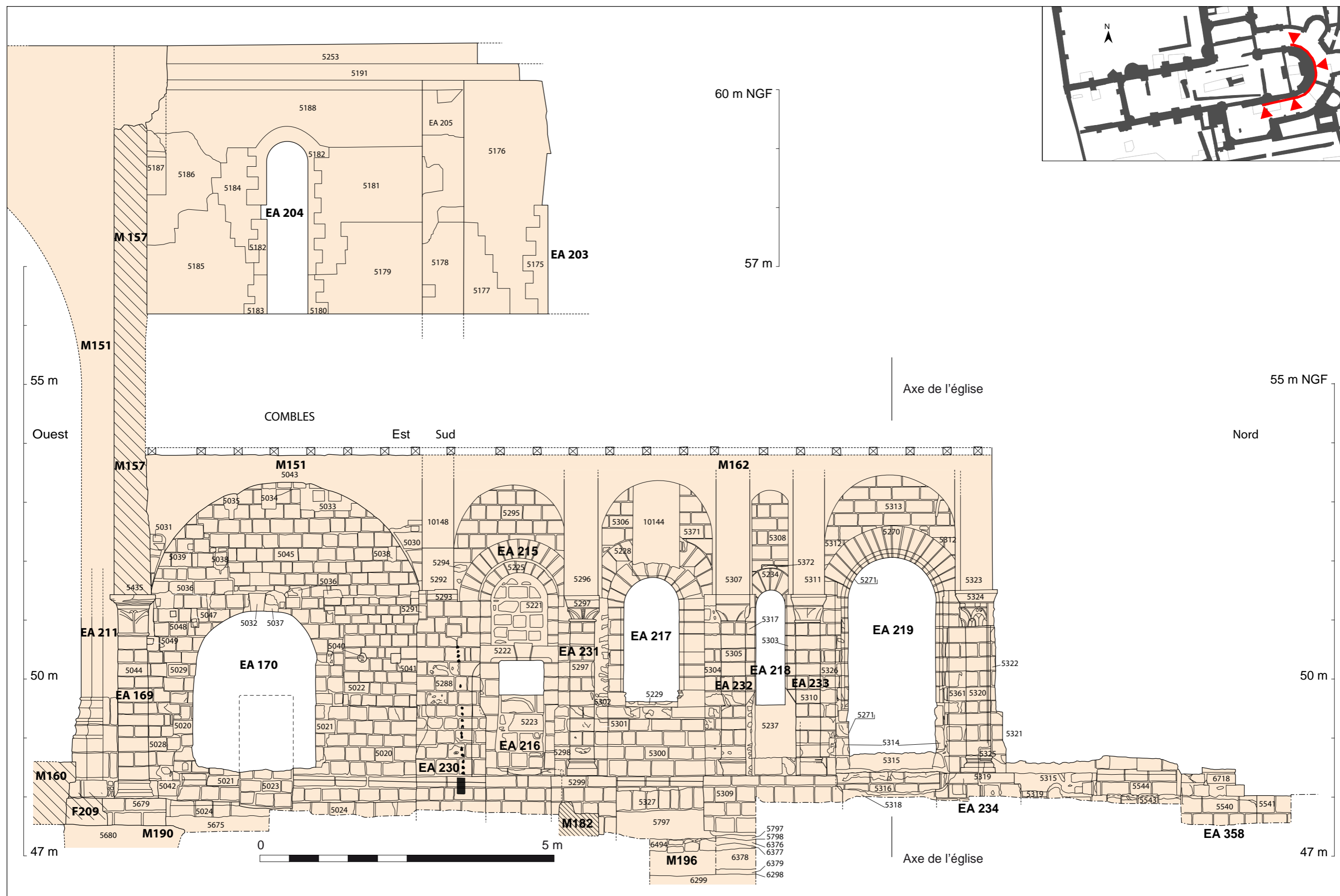
Planche 23 : relevé de l'élévation extérieure de la travée droite de chœur et du rond-point du chœur (pour le relevé phasé, voir figure 23)
