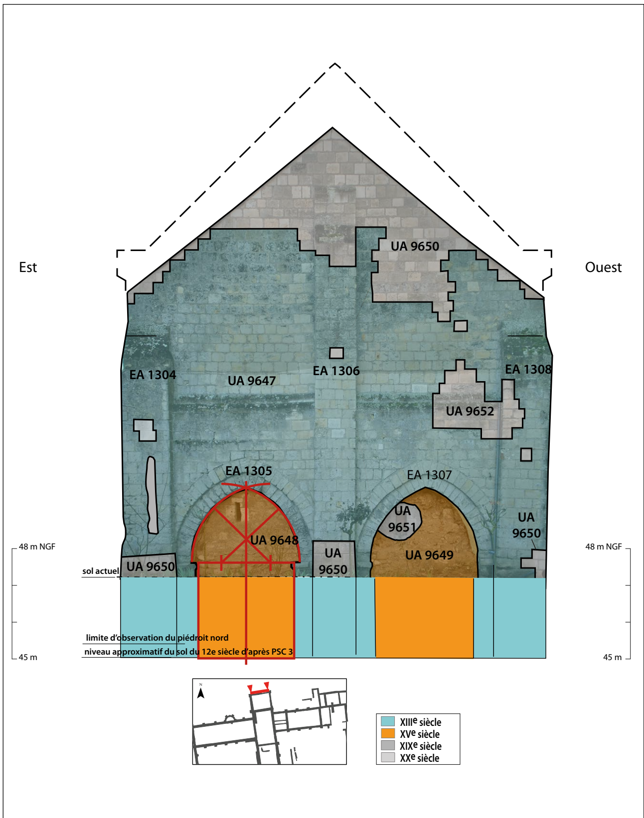
Figure 41 : analyse du bâti du pignon du présumé garage à bateaux (vue du nord – photo redressée : Frédéric Epaud (LAT) et Julien Noblet)
