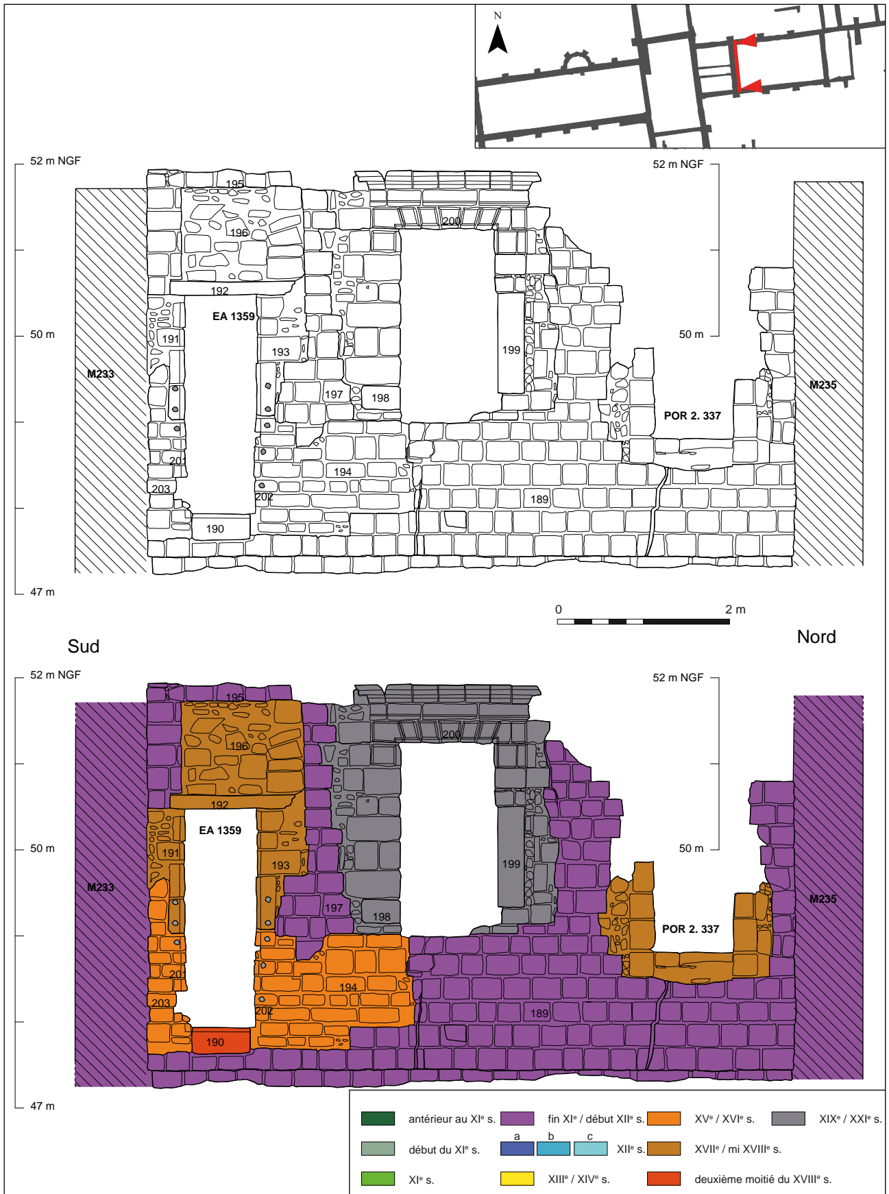
Figure 49 : analyse du bâti du mur pignon occidental du « régulier », côté intérieur (M 237) (d'après le relevé de Bancaud, Body 2006)
