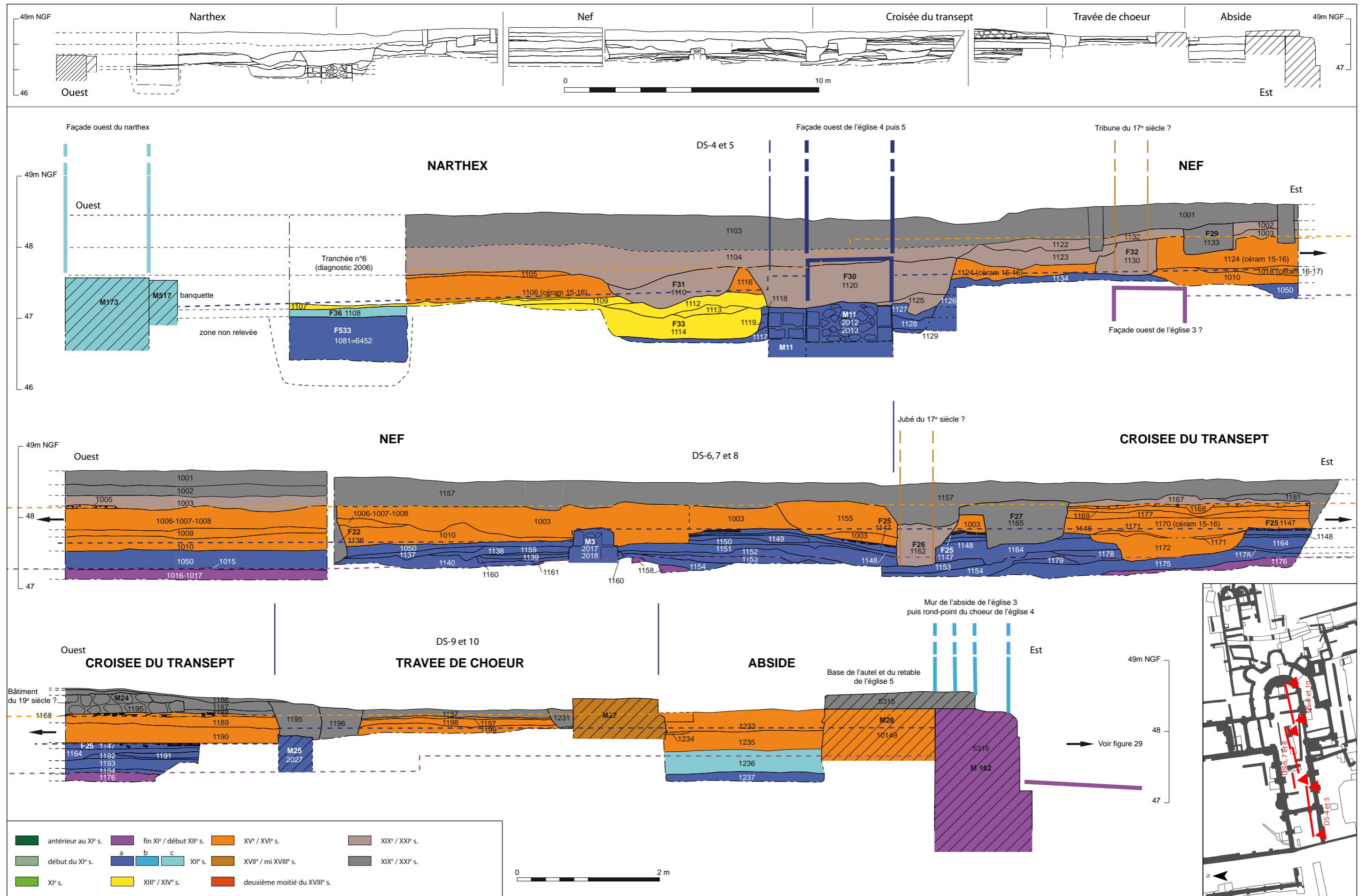
Planche 26 : coupe stratigraphique des sols dans l'axe de l'église (relevé de la tranchée n°4 réalisée lors du diagnostic de 2006)
