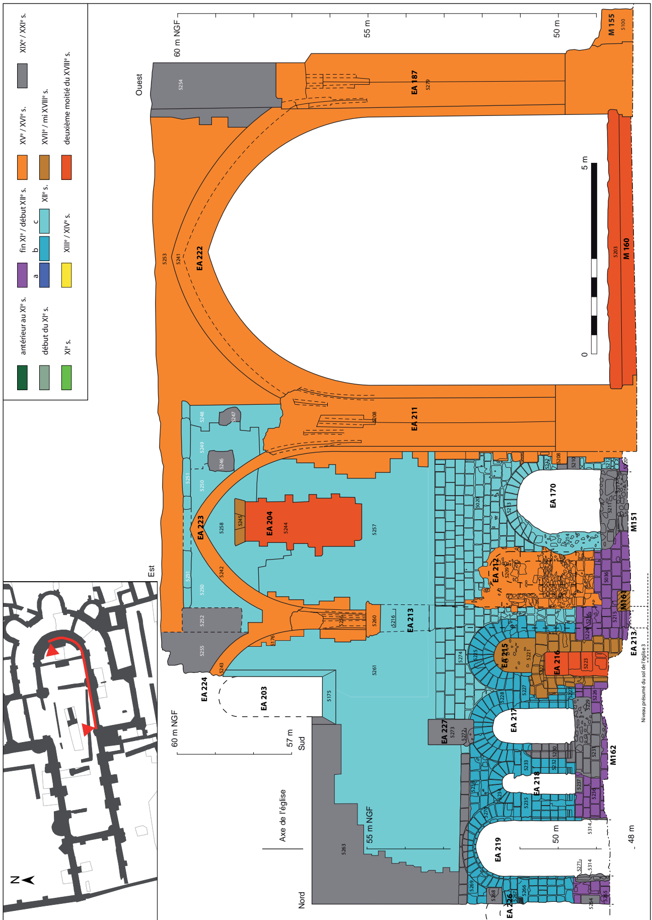
Figure 23 bis : relevé phasé de l'élévation intérieure du mur sud du chœur de l'église et de l'arc du transept sud (pour le relevé non phasé, voir planche 24)
