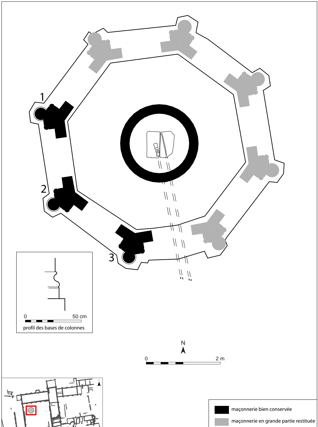
Figure 46 : plan des vestiges du lavabo du cloître
