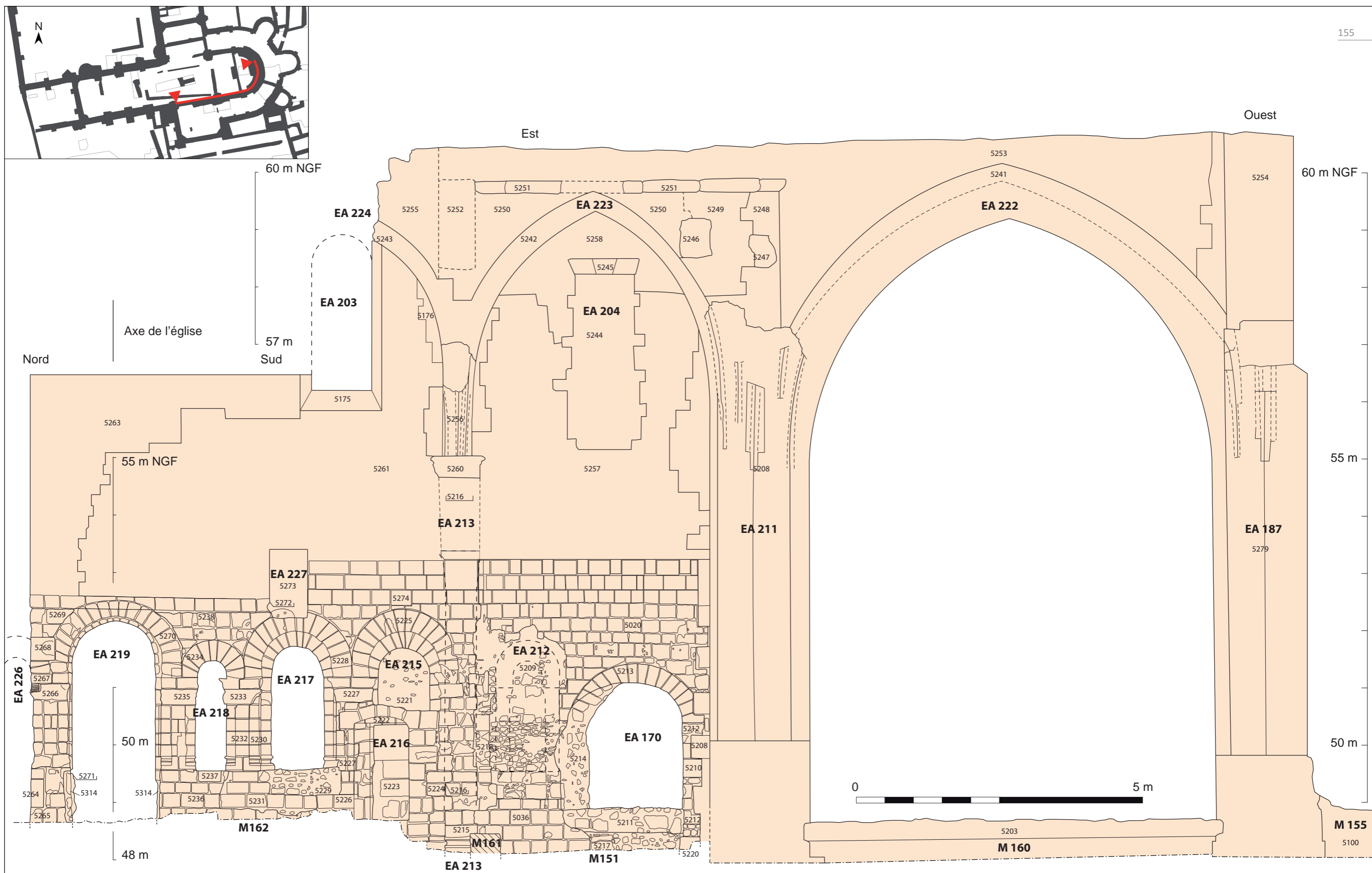
Planche 24 : relevé de l'élévation intérieure du mur sud du chœur de l'église et de l'arc du transept sud (pour le relevé phasé, voir figure 23 bis)
