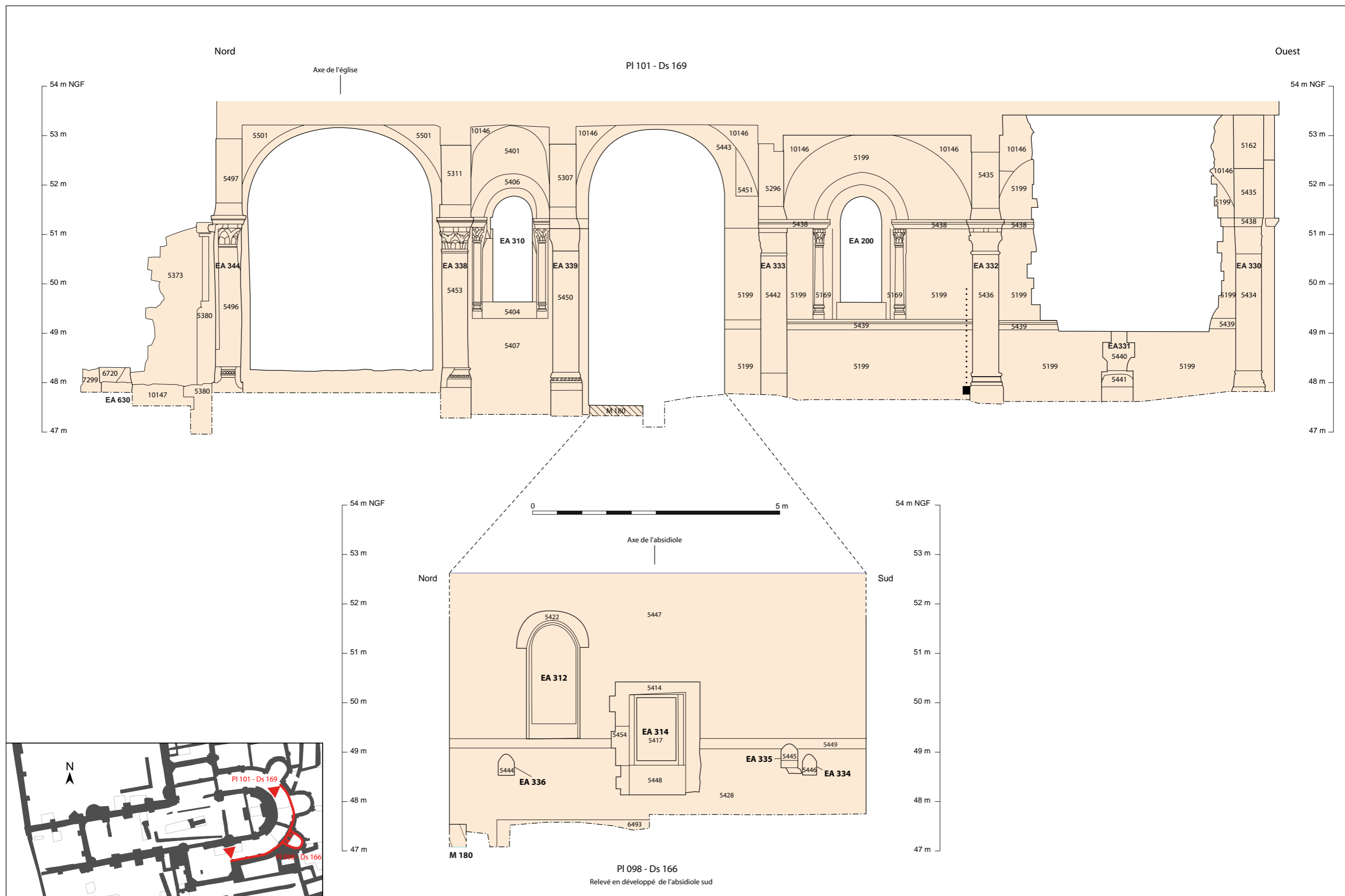
Planche 25 : relevé de l'élévation du mur extérieur du déambulatoire (face interne) et relevé développé de la face interne de la chapelle sud-ouest du déambulatoire (pour le relevé phasé, voir figure 28)
