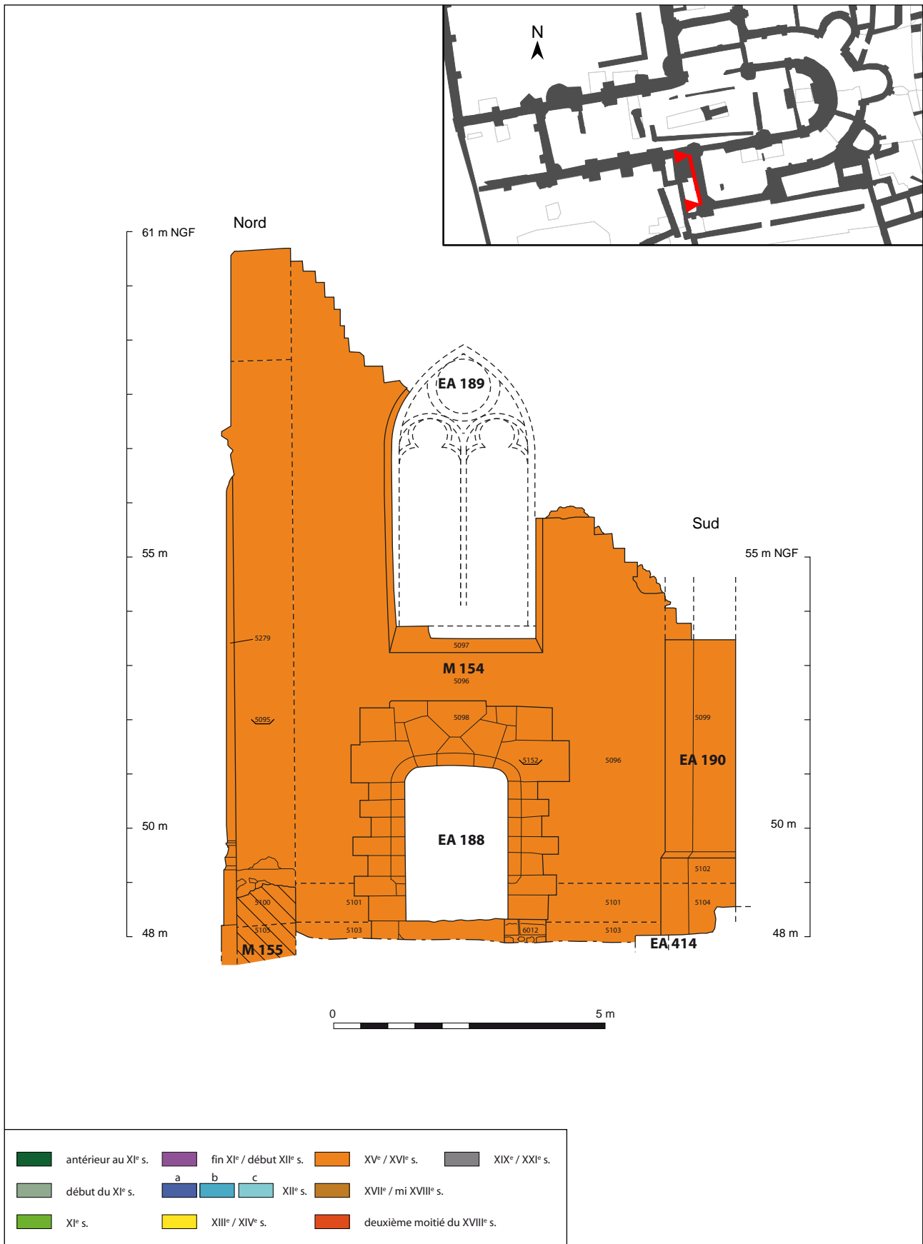
Figure 63 : élévation extérieure phasée du mur ouest du transept sud de l'église n°5, avec restitution du remplage de la baie
