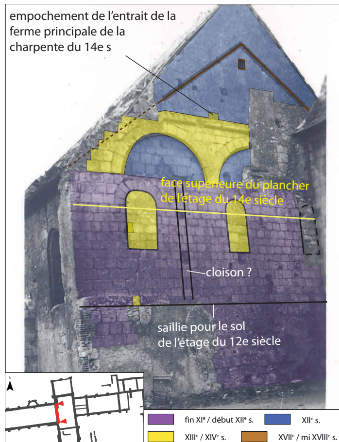
Figure 40 : analyse du bâti du parement interne du mur gouttereau ouest de l'aile orientale du carré claustral, à partir d'une photo prise en 1948 avant restauration du bâtiment (vue de l'ouest)
