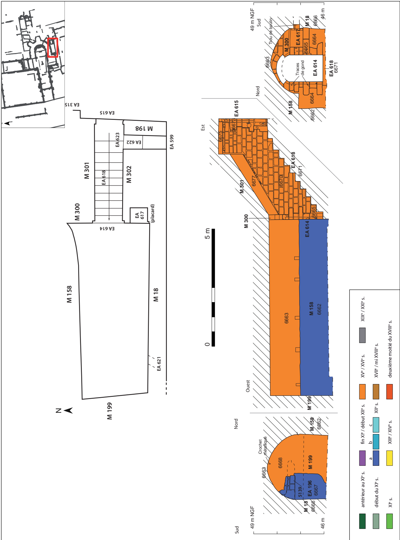
Figure 59 : plan, coupes et élévations de la cave du logis du sacristain, jouxtant l'église au sud
