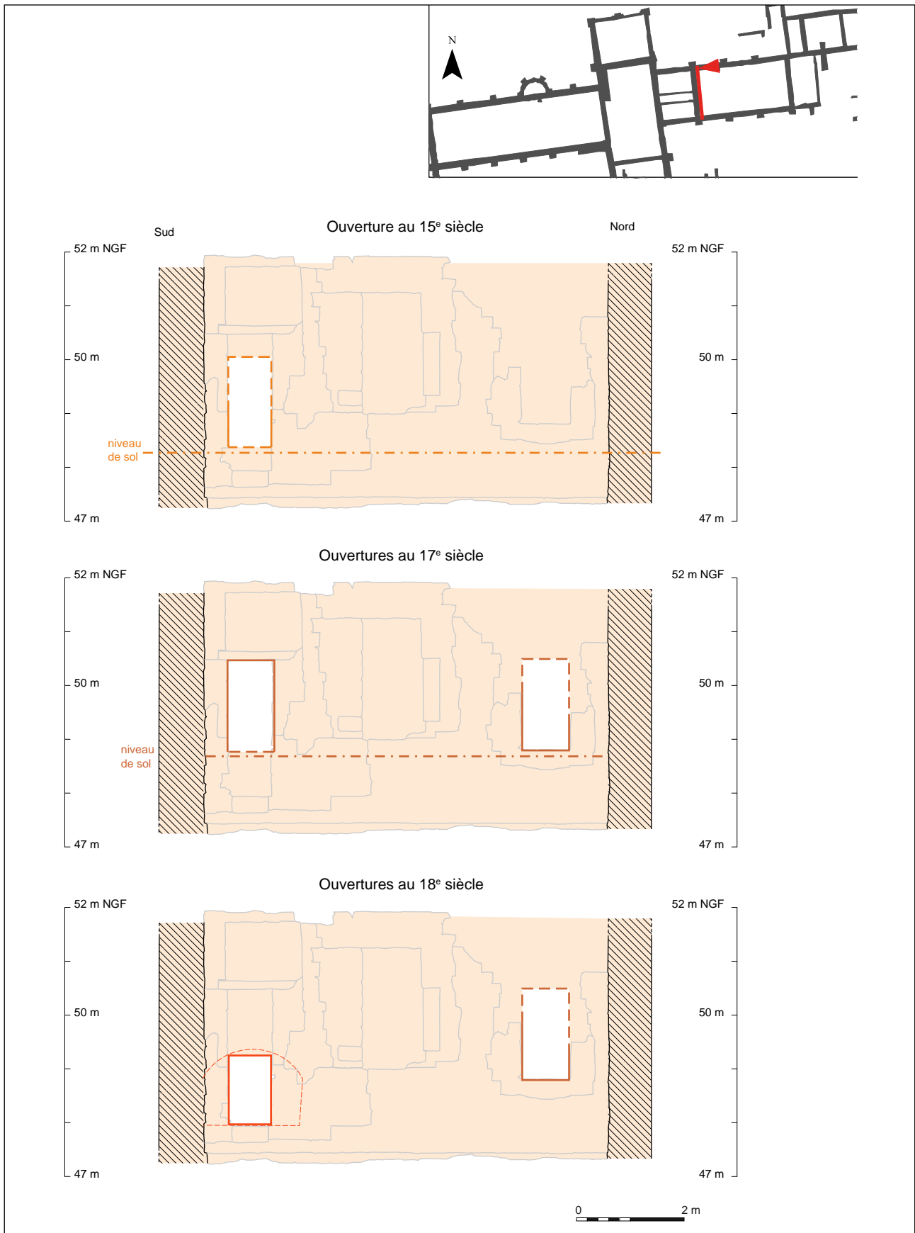
Figure 49 bis : analyse des ouvertures dans le du mur pignon occidental du « régulier » (M 237)
