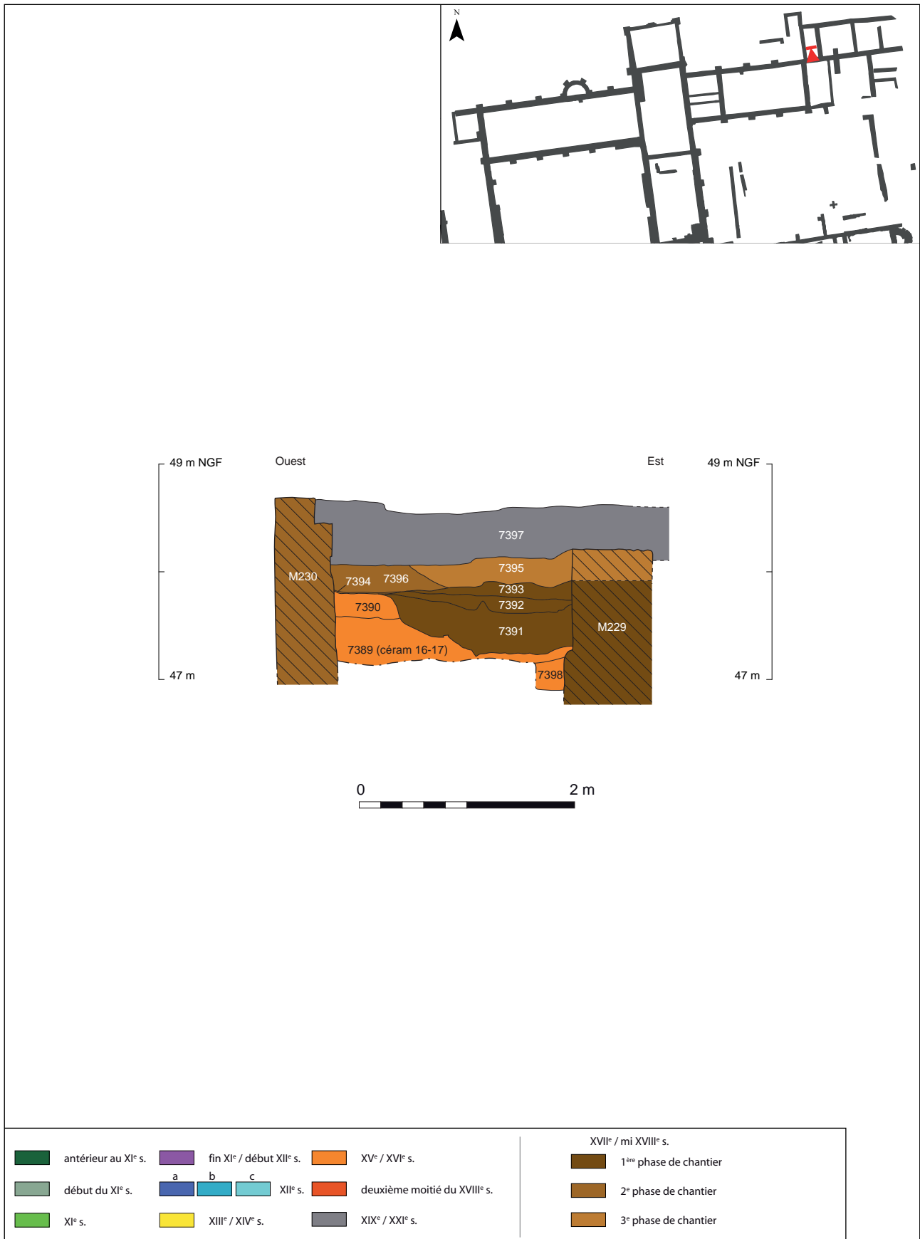
Figure 66 : coupe nord du sondage n°35, sur le sous-prieuré
