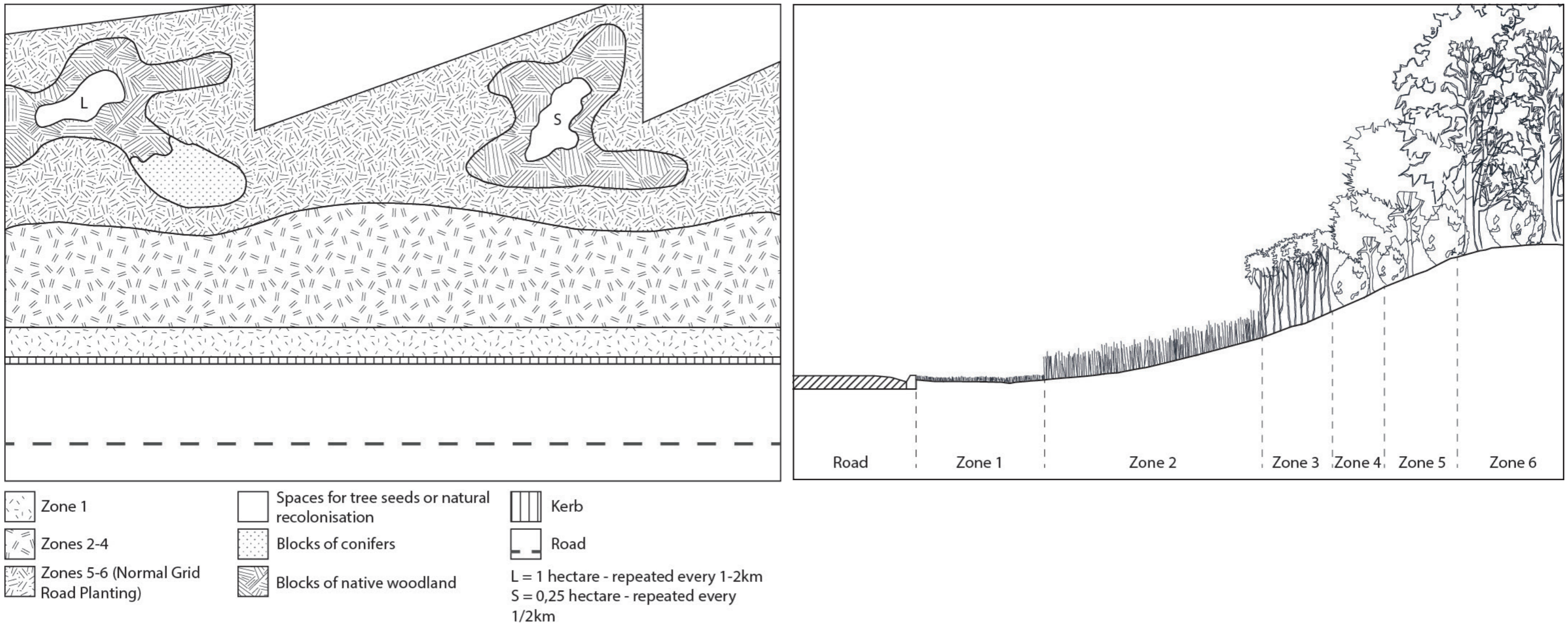
Plan de l'aménagement des bords de routes. Source: Kelcey and MKDC, 1974. Redessin M. Forget.
