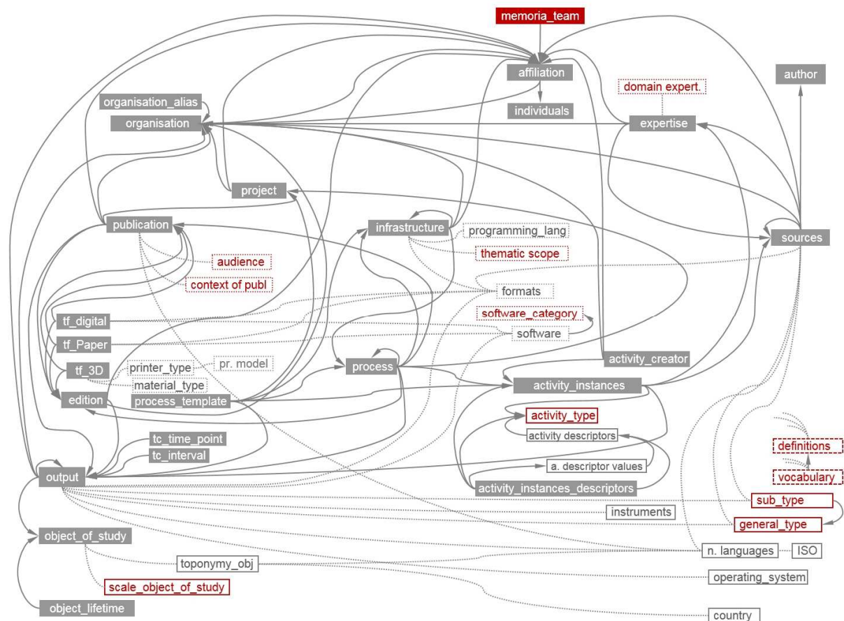
Figure 3 : Schéma de la base de données, en rouge les tables à interroger
