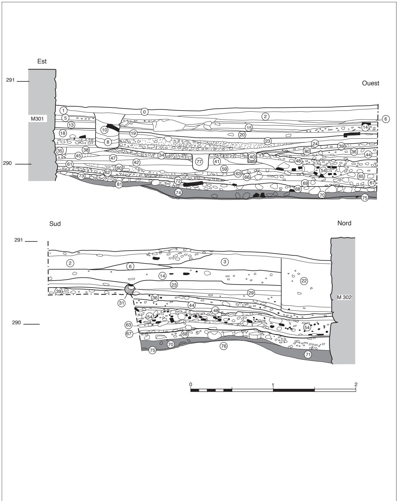
Ill. annexe 23. Lyon, les contextes précoces des fouilles du « sanctuaire de Cybèle ». Horizon IA, sondage D1 : coupe stratigraphique est-ouest et nord-sud. En grisé, le remblai antérieur au premier niveau de rue (68-73).
