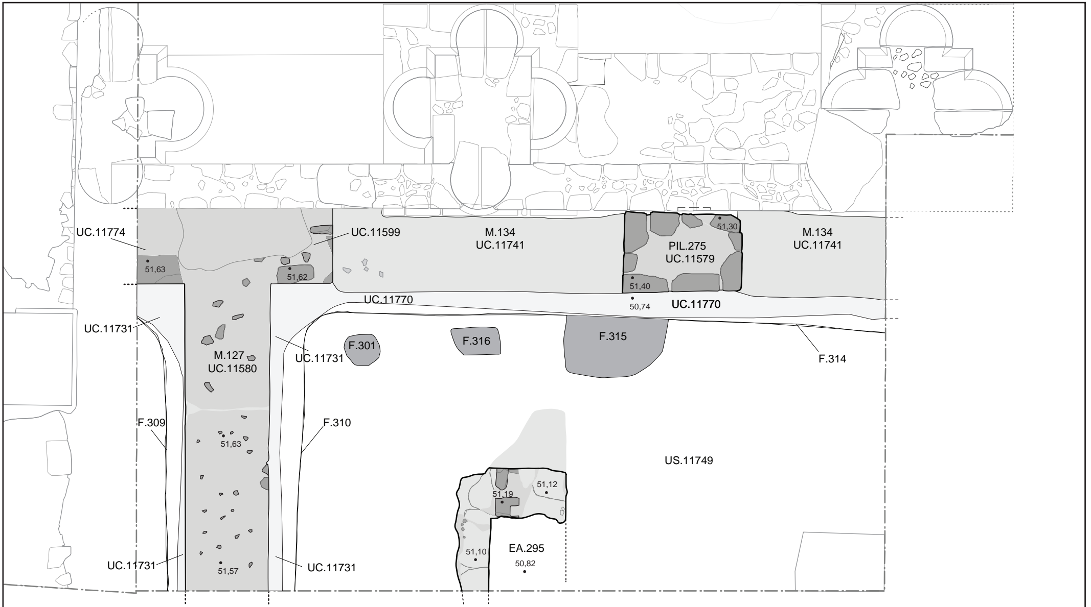
Tours site 17 - Marmoutier 2014 Fig. 7 Zone 1, Secteur 7 Plan des structures en fondation de l'église des environs de l'an mil.
