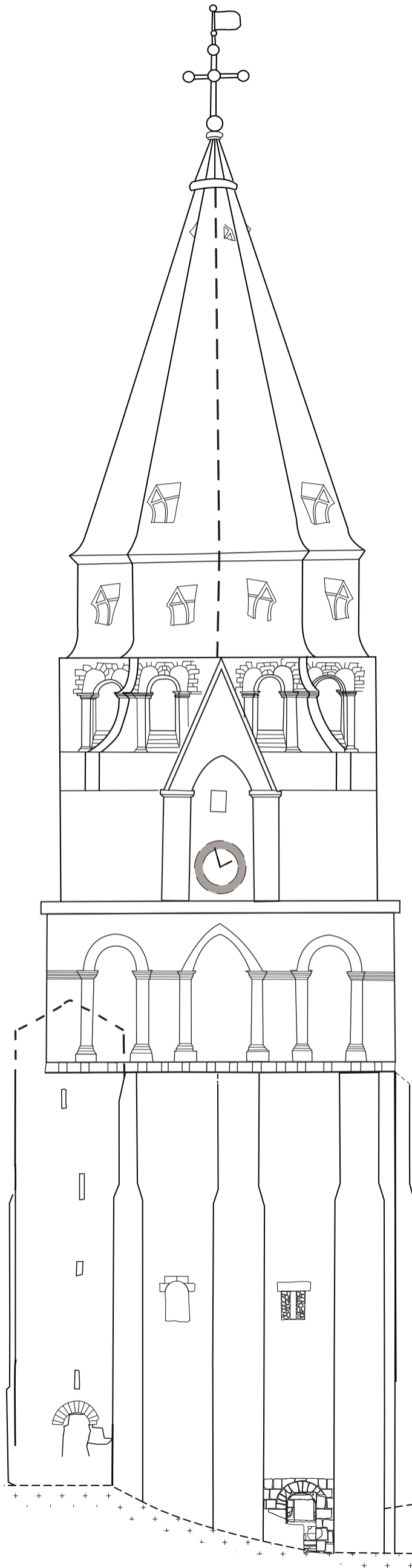
Tours site 17 - Marmoutier 2014 0 5 10 m Fig. 27 Zone 5 Proposition de restitution de l'élévation de la façade sud de la tour des cloches.
