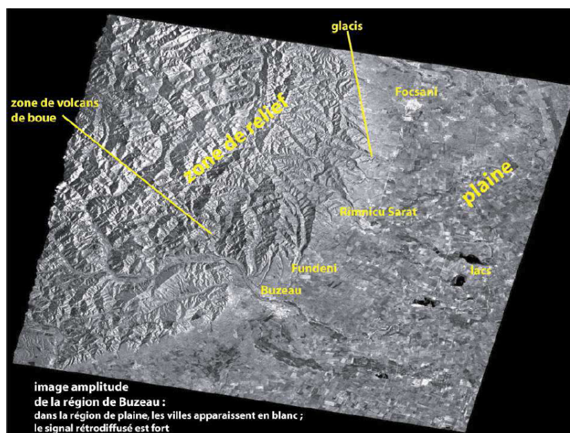
FIGURE 5 – Image radar d'amplitude géoréférencée de la zone d'étude. Georeferenced radar amplitude image of the study area.
