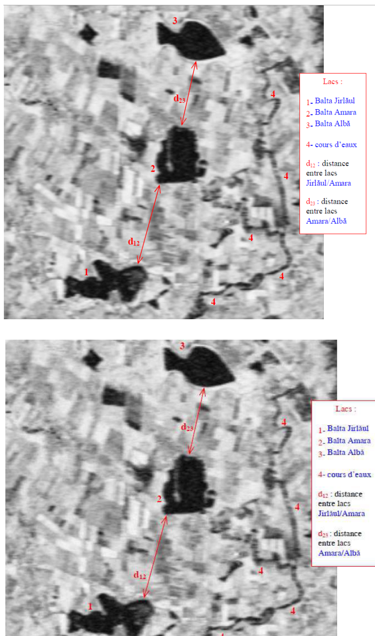
FIGURE 3 – Zone des lacs dans l'image de cohérence (couple tandem, 28/29 mai 1995), Les lacs sont numérotés de plus proche de la ville de Buzău.
