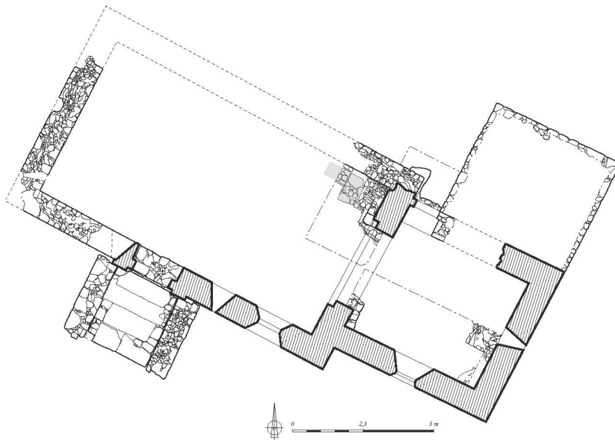
1 - Saint-André-des-Eaux, plan de l'église, en grisé la maçonnerie antérieure (cl. M. Dupuis).
