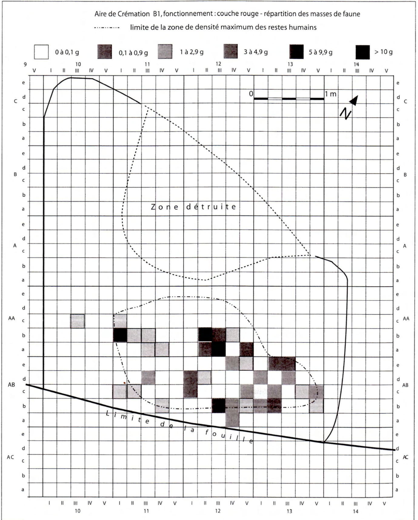
Fig. 124. Répartition des restes fauniques de la couche rouge (US17132) de l'aire de crémation B1 en fonction de leur masse.
