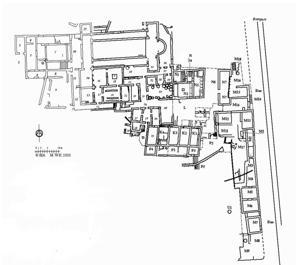
Fig. 1 - Byllis, plan schématique de la cathédrale et du quartier épiscopal : implantation des fouilles et nettoyages en 2010 (dessin M. Wurch-Kozelj).
