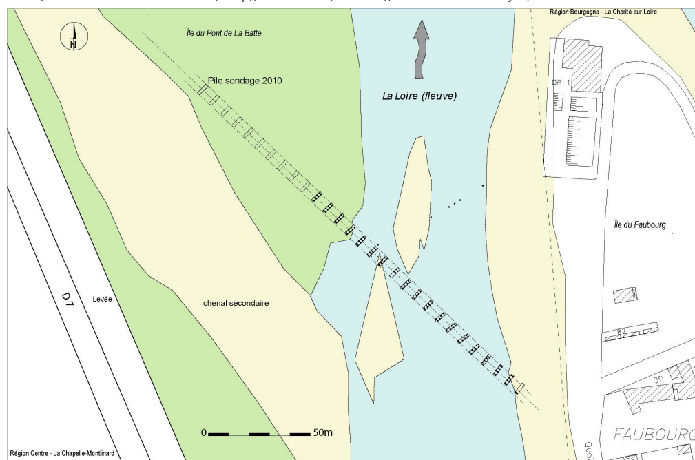
Fig. 1 - Plan des vestiges du pont du XIII e siècle découvert dans la Loire entre La Chapelle-Montlinard et La Charité-sur-Loire (relevé de terrain S. Couteau (Inrap), G. Lemaire (DRASSM), A. Dumont et P. Moyat).
