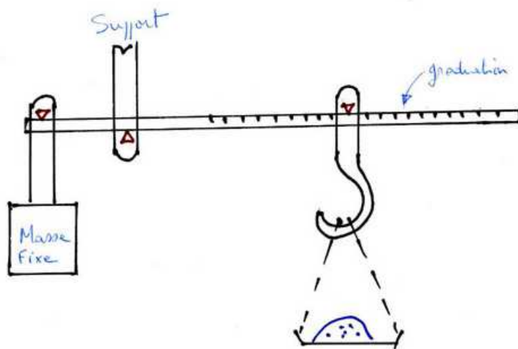
FIG. 24 – Balance romaine
