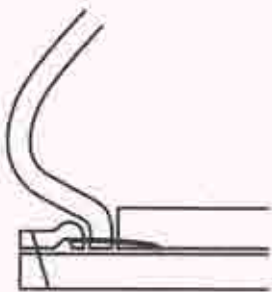
Fig. 2 : vue en coupe du semelage cousu petit point.
