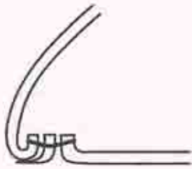
Fig. 1 : vue en coupe du semelage cousu retourné.
