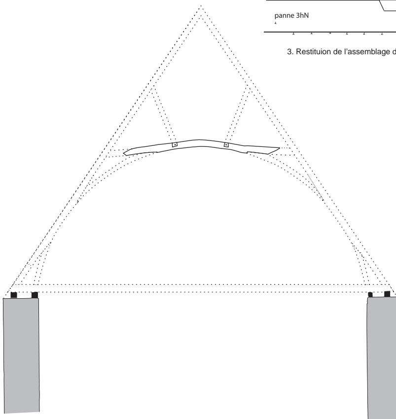
4. Restituiou d'une ferme complète à partir d'un entrait retroussé.
