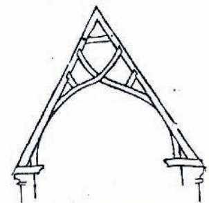
5. Entrait retroussé réemployé comme chevron dans la charpente actuelle. les deux entailles à mi-bois sont bien visibles.
