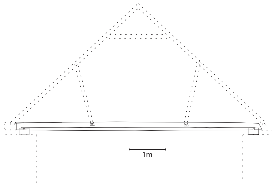
5. restitution d'une ferme de type romane à partir de l'entrait et d'une partie de chevron
