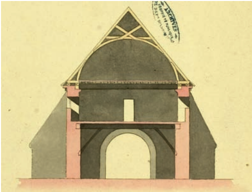
3. coupe des Grandes Ecuries réalisées par Pinguet en 1809 ADIL, cote V10_1_13
