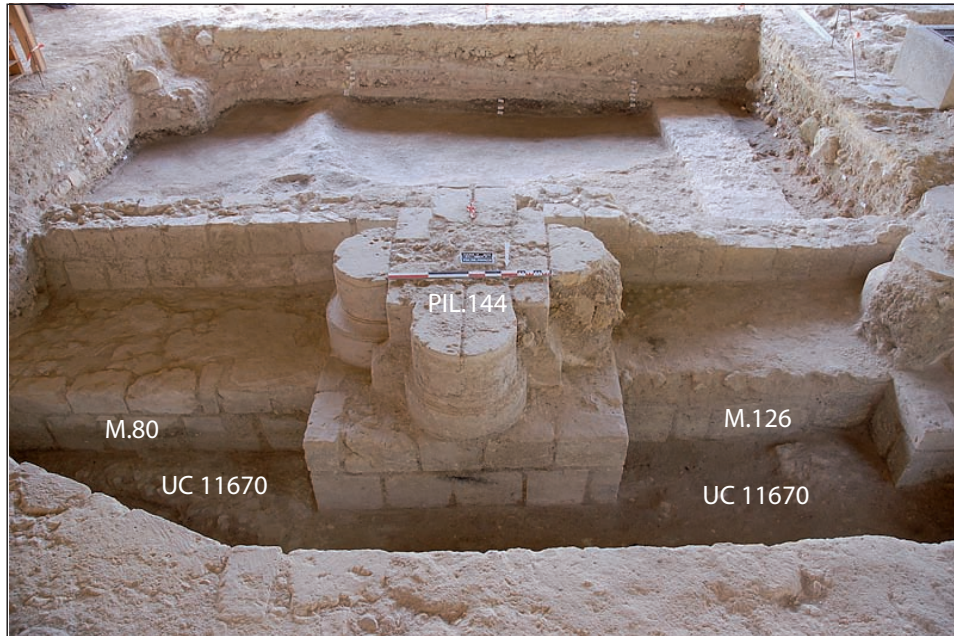
Fondations et élévation de la pile 144 vues depuis le nord
