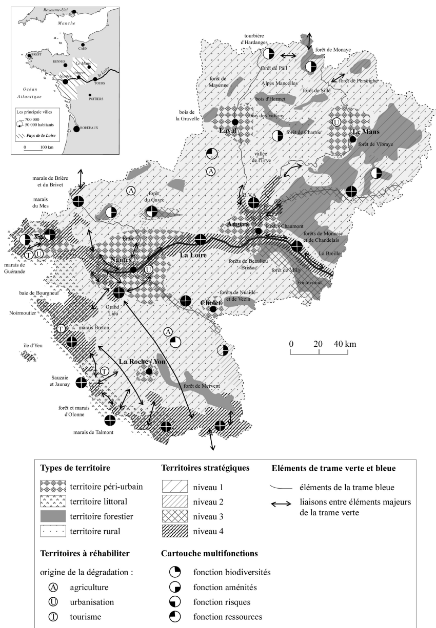
Figure 1 Carte de synthèse des services des espaces ruraux dans les Pays de la Loire ; l'aménité paysagère (le paysage d'agrément) est aujourd'hui reconnue comme une des fonctions de l'espace rural.
