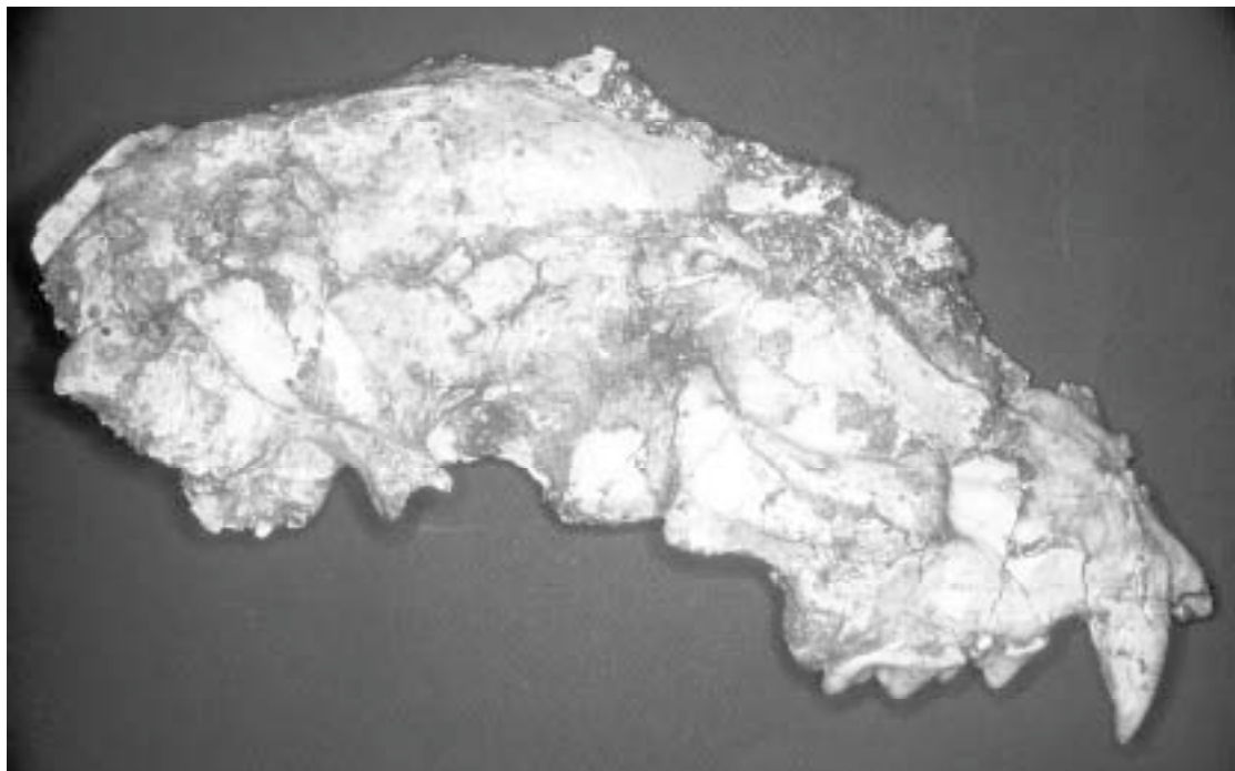
Photo 6 : Casablanca, Ahl Al Oughlam, crâne d' Acynonix aicha , une nouvelle espèce fossile de guépard (© D. Geraads).
