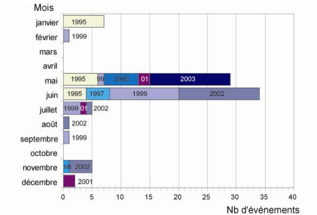
Figure 3.8 : Répartition annuelle des coulées boueuses pour le Haut-Rhin entre 1995 et 2003 (Dossiers d'indemnisation au titre de catastrophes naturelles – Préfecture 68)
