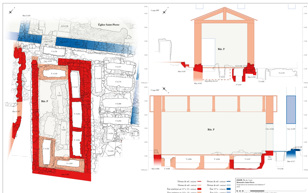
Fig. 8 - Saint-Pierre d'Osor, plan et coupes restituées du mausolée.
