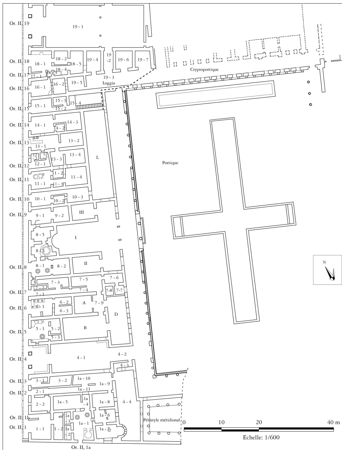
Fig. 1. Nomenclature des pièces de l' Insula Orientalis II a (DAO N. Monteix, d'après relevé F. Ferrajoli modifié par L. Trinca et M.R. Acetosio).
