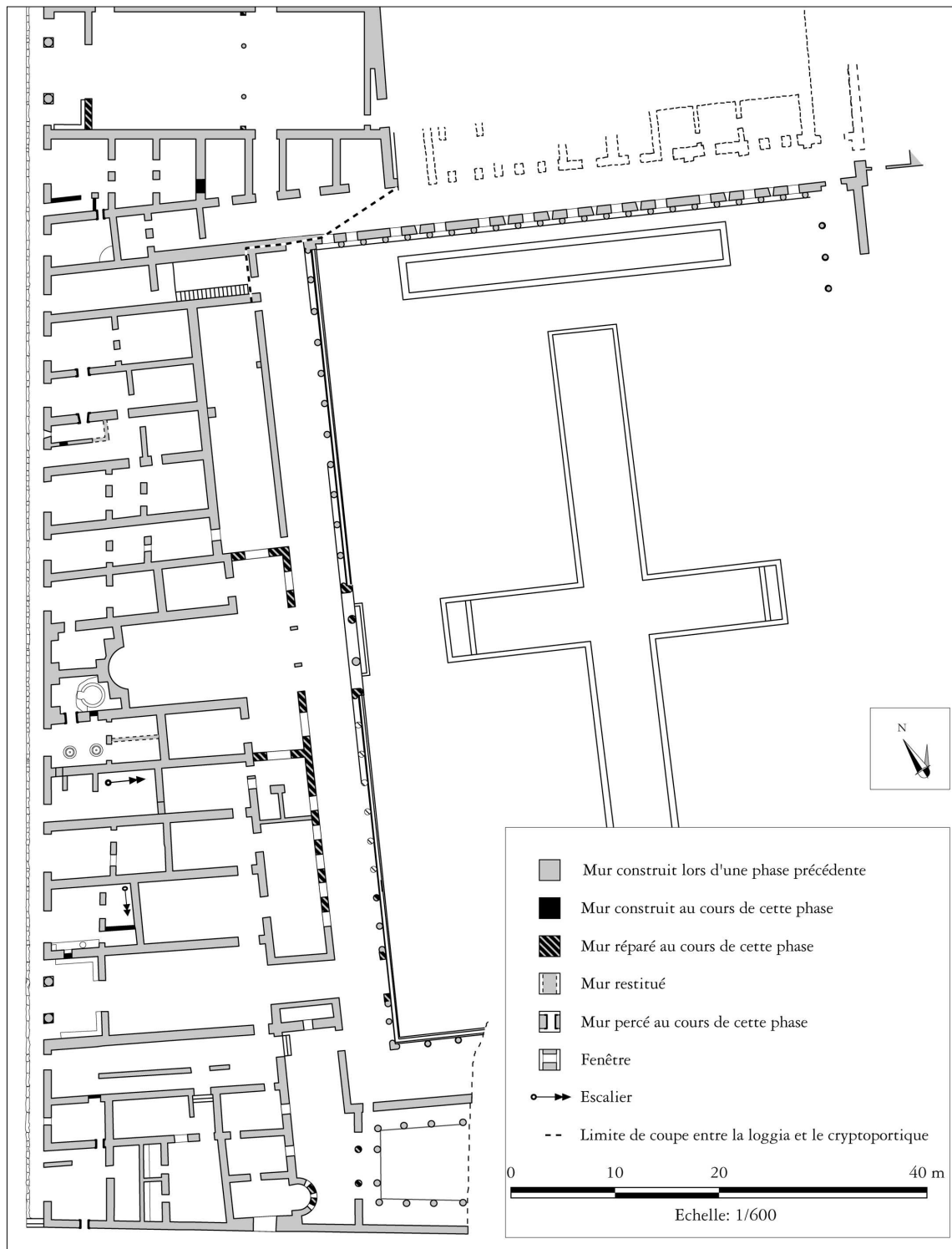
Fig. 16. Restitution du plan de la seconde phase de l' Insula Orientalis II a entre le séisme de 62 et celui du début des années 70 (DAO N. Monteix, d'après relevé F. Ferrajoli modifié par L. Trinca et M.R. Acetoso).
