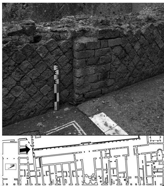
Fig. 9. Pièce 19-3 de la loggia , mur sud. La césure verticale visible dans la maçonnerie originelle montre que les niveaux de circulation situés au-dessus de l'extrados du cryptoportique se s'appuient sur les constructions constituant l'angle nord-ouest de l'édifice.
