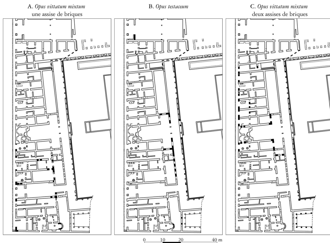
Fig. 5. Répartition des différents types d'appareils mis en œuvre dans l'Insula Orientalis II e . A. Opus vittatum à un rang de briques. B. Opus testaceum . C. Opus vittatum à deux rangs de briques (DAO N. Monteix).
