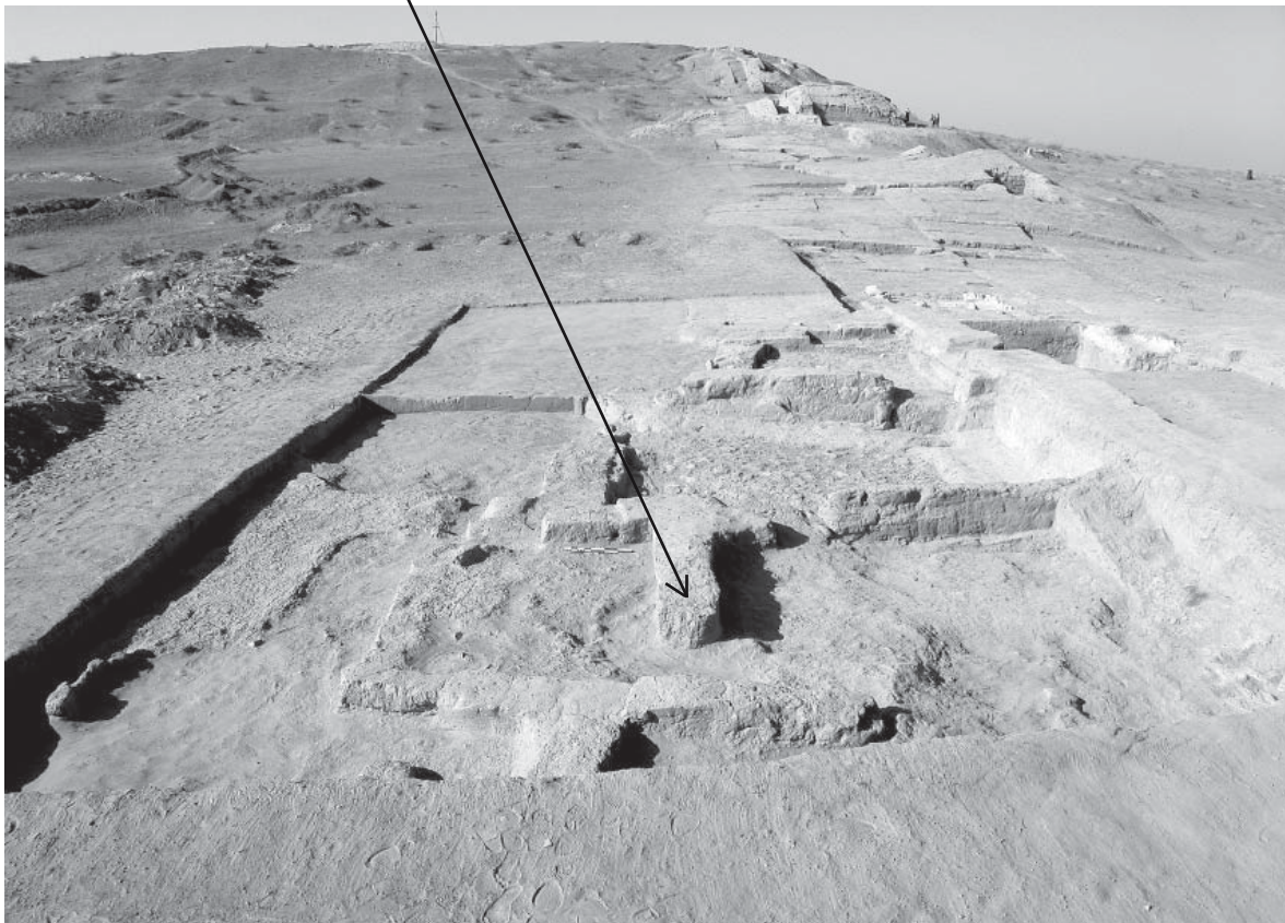
Fig. 23 - Tchingiz Tepe. Le sondage contre la cortina C6-7, occupation civile ou religieuse contre la muraille. Vue vers le nord.
