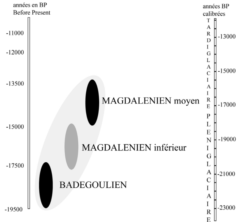
Figure 12 - Répartition chronologique du Badegoulien et des premières phases du Magdalénien selon les dates radiocarbones (C14)
