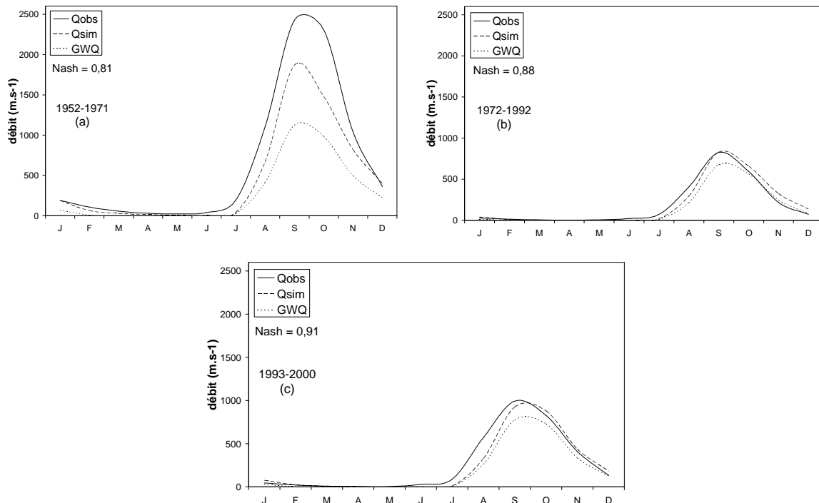
Fig. 3 Moyennes mensuelles des débits mesurés Q_{obs} et simulés Q_{sim} , et des débits de base simulés GWQ (générés par les nappes souterraines) à Douna : (a) 1952-1971; (b) 1972-1992 ; (c) 1993-2000.
