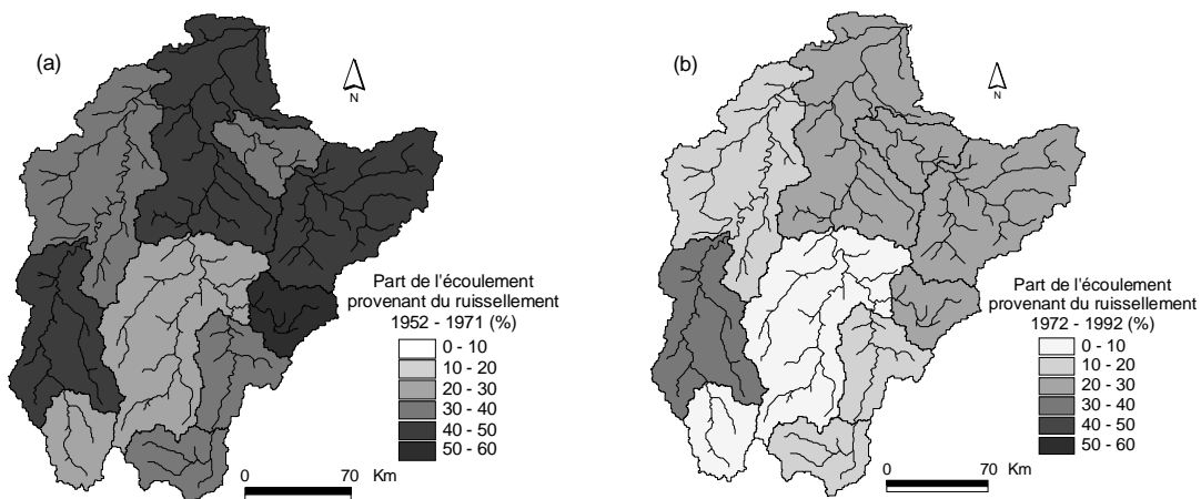
Fig. 5 Estimation de la part de l'écoulement provenant du ruissellement : (a) moyenne 1952-1971; (b) moyenne 1972 -1992.
