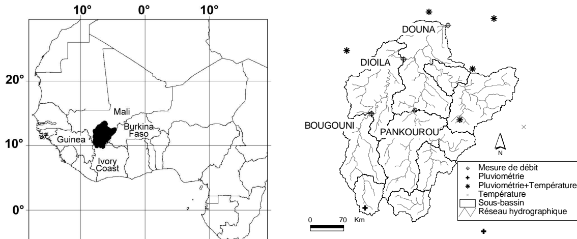
Fig. 1 (a) Localisation du bassin du Bani (b) Stations de mesure.
