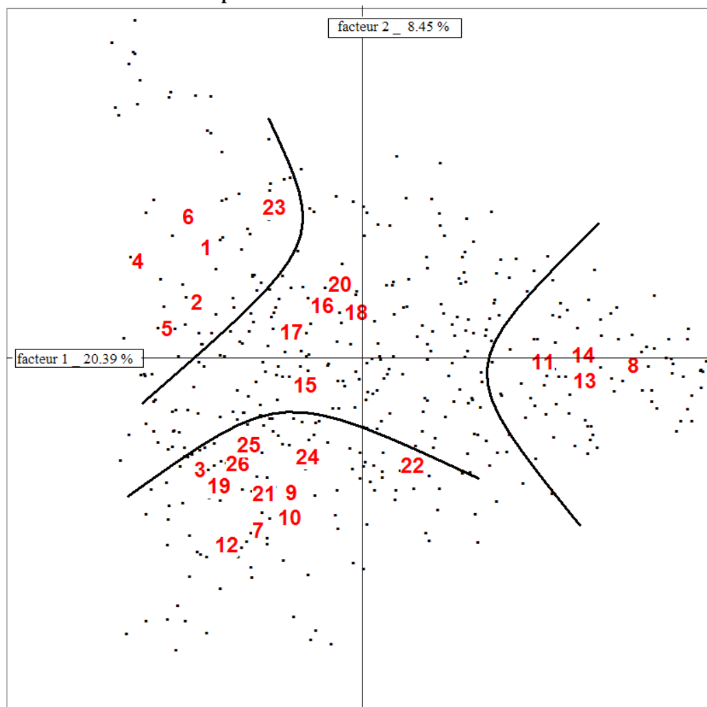
Graphe de la AFC Macro-distribution 215 × 26 textes
