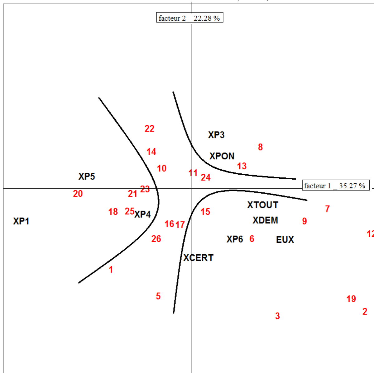
AFC Macro-distribution 215 x 26 textes (sans Tu)
