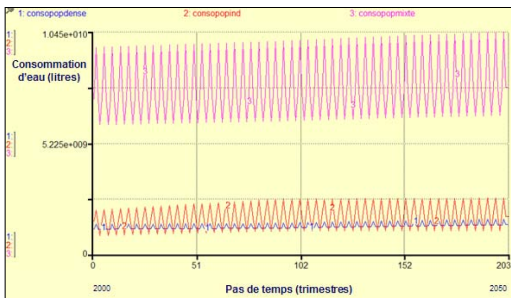
Figure 3: Résultats des simulations du modèle « avec interventions »
