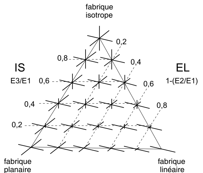
Fig. 6 - Diagramme de Benn
