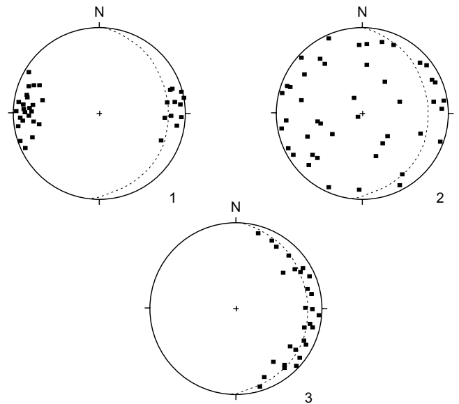
Fig. 4 - Diagrammes de Schmidt. 1 – fabrique linéaire (les points représentatifs des axes sont groupés autour d'une direction), 2 – fabrique isotrope (les points sont dispersés), 3 – fabrique planaire (les points se regroupent sur un plan indiqué par le trait pointillé)
