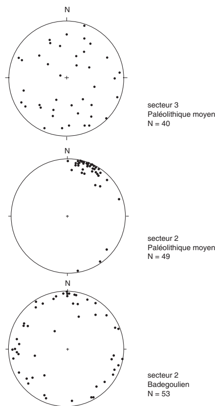
Fig. 11 - Fabriques relevées sur le site de Croix-de-Canard, diagrammes de Schmidt
