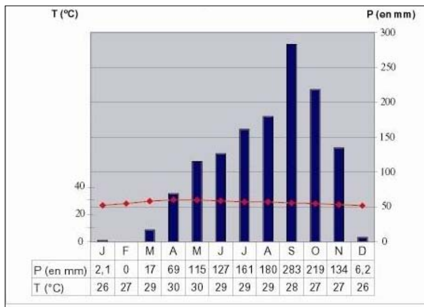
Fig. 5 — Diagramme ombrothermique de Phnom Penh (avec P = 2T ) – Station de Pochentong, 1985-1997 (D'après JICA, 1999. Réalisation : C. Pierdet)
