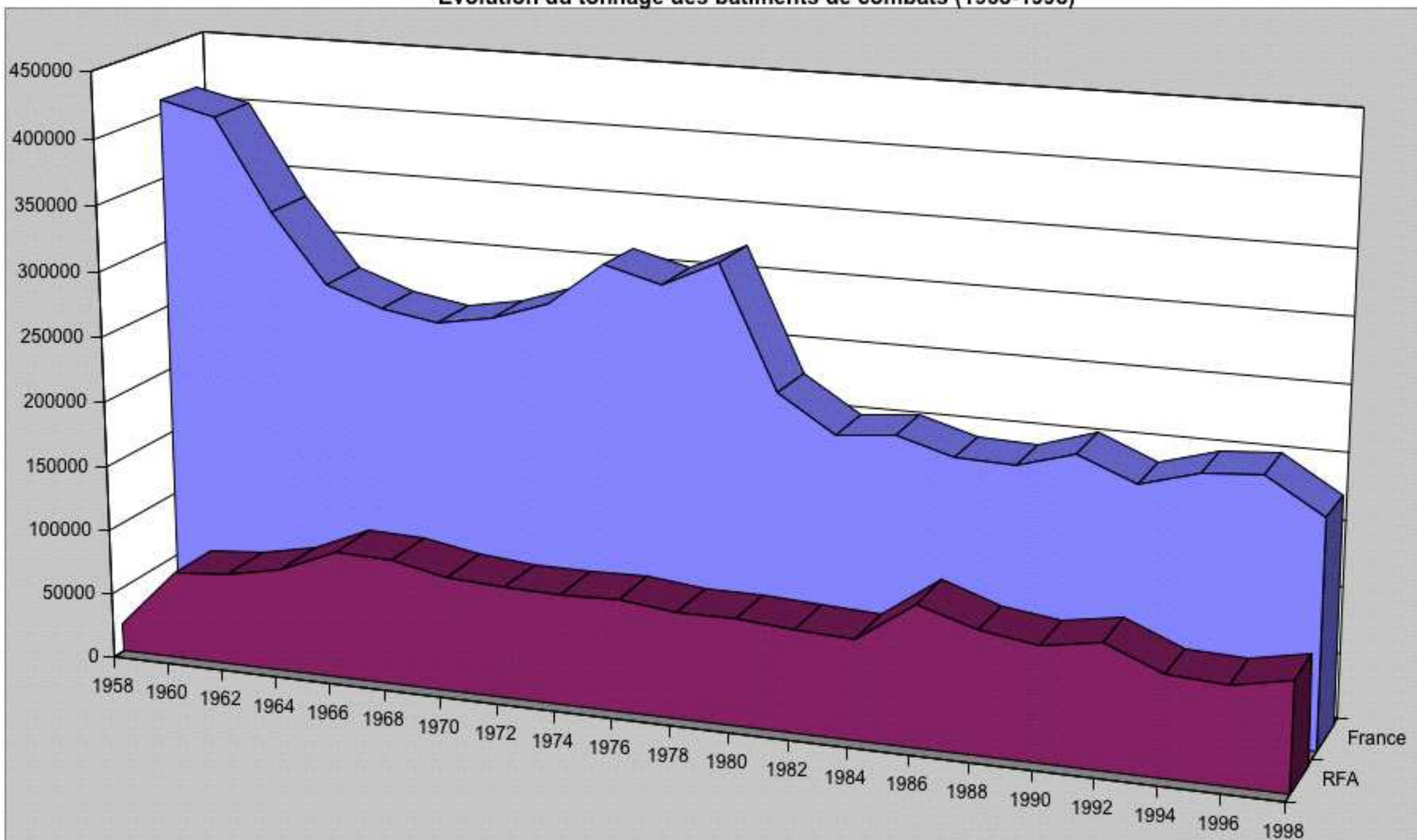
Graphique n° 2 : France - R.F.A. Evolution du tonnage des bâtiments de combats (1958-1998)
