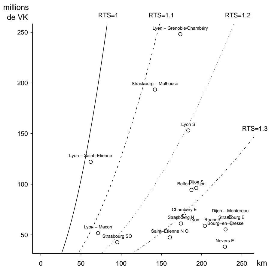
FIG. 1 – Nomogramme des rendements de taille pour les sous-réseaux : trafic en fonction de la longueur de lignes.
