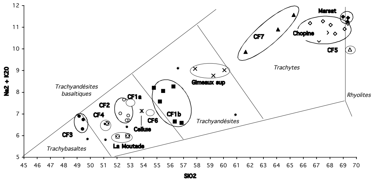
Figure 1 : Composition chimique des différents téphras reconnus dans un diagramme SiO_2/Na_2O+K_2O (Le Bas et al. , 1985) Chemical composition of identified tephra in SiO_2/Na_2O+K_2O (weight%) diagram (after Le Bas et al. , 1985).
